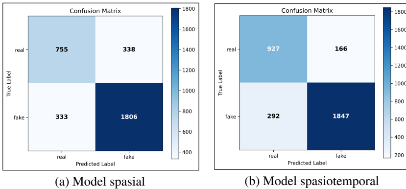
Gambar 4.6 Confusion matrix pada eksperimen baseline .
