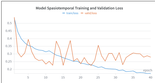
Gambar 4.8 Kurva training loss dan validation loss pada eksperimen epoch maksimum 40 untuk model spasiotemporal.
