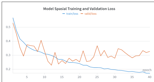
Gambar 4.7 Kurva training loss dan validation loss pada eksperimen epoch maksimum 40 untuk model spasial.
