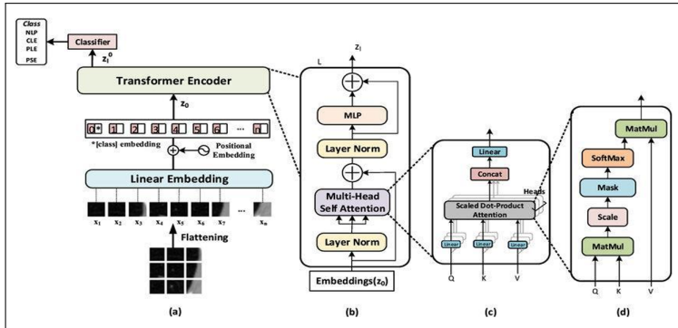
Gambar 2.2 Arsitektur Vision Transformer (ViT). Sumber: Dosovitskiy et al. [6]
