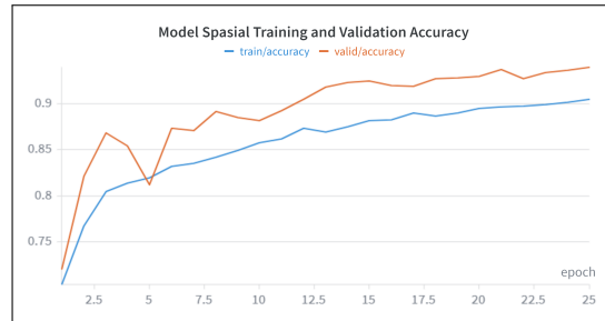
Gambar 4.4 Kurva training accuracy dan validation accuracy pada eksperimen baseline untuk model spasial.
