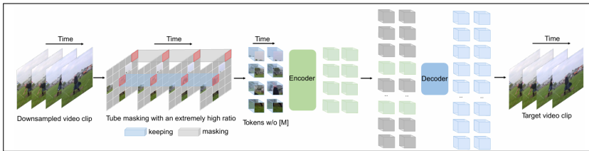
Gambar 2.3 Arsitektur VideoMAE dengan Asymmetric Encoder-Decoder dan Tube Masking. Sumber: Tong et al. [11]
