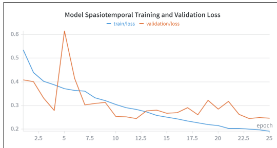
Gambar 4.3 Kurva training loss dan validation loss pada eksperimen baseline untuk model spatiotemporal.
