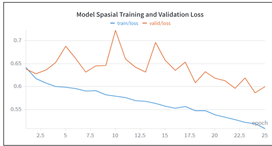
Gambar 4.9 Kurva training loss dan validation loss pada eksperimen learning rate 5e-4 untuk model spasial.
