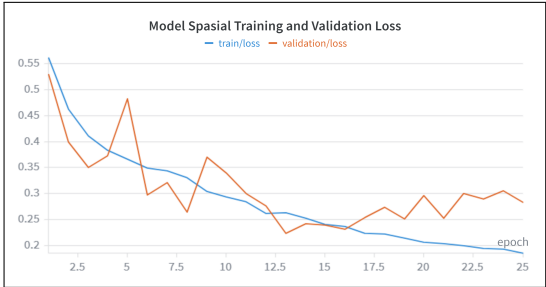
Gambar 4.2 Kurva training loss dan validation loss pada eksperimen baseline untuk model spasial.
