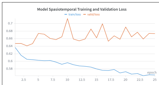
Gambar 4.10 Kurva training loss dan validation loss pada eksperimen learning rate 5e-4 untuk model spasiotemporal.
