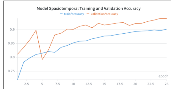
Gambar 4.5 Kurva training accuracy dan validation accuracy pada eksperimen baseline untuk model spasiotemporal.
