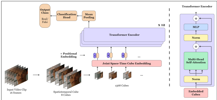
Gambar 3.10 Arsitektur model spasiotemporal berbasis VideoMAE untuk klasifikasi deepfake
