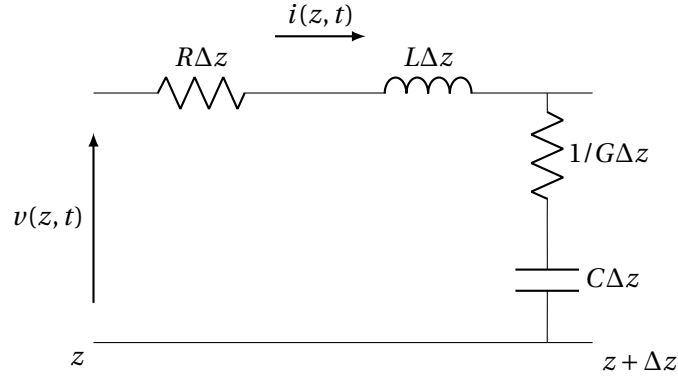
Figura 6.1. Circuito de parámetros concentrados equivalente a un segmento de línea de longitud \Delta z . La línea completa es la cascada de infinitos segmentos de este tipo.
