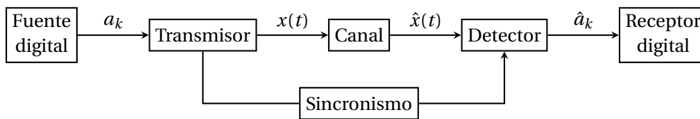
Figura 3.1. Esquema de un sistema de modulación digital.
