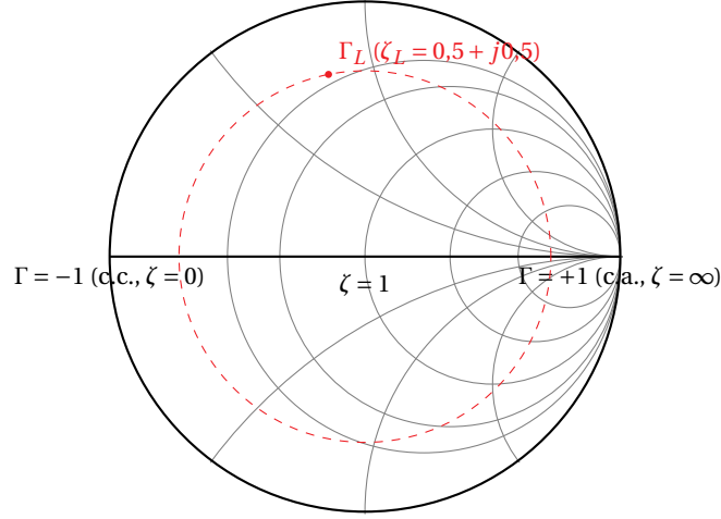
Figura 6.2. Esquema de la Carta de Smith: disco |\Gamma| \leq 1 con la grilla de resistencia normalizada r constante (circunferencias tangentes al punto \Gamma = 1 ) y reactancia normalizada x constante (arcos). Moverse a lo largo de la línea es rotar sobre la circunferencia punteada (ROE constante) que pasa por \Gamma_L .
