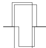
Figura 3.9. Ejemplos de diagrama de ojo para pulsos polares RZ
