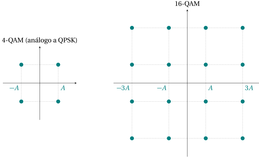
Figura 5.5. Constelaciones QAM.
