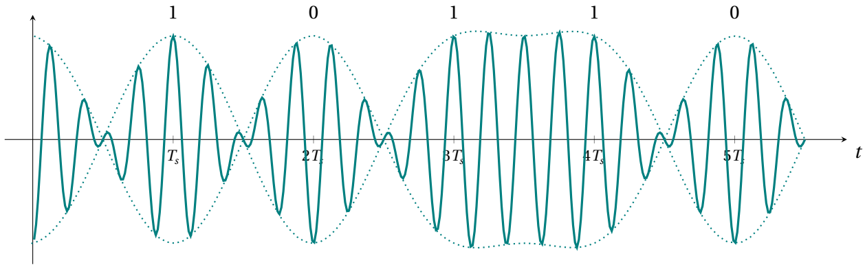
Figura 5.2. Onda BPSK con pulsos de Nyquist de exceso de ancho de banda \alpha = 1 .
