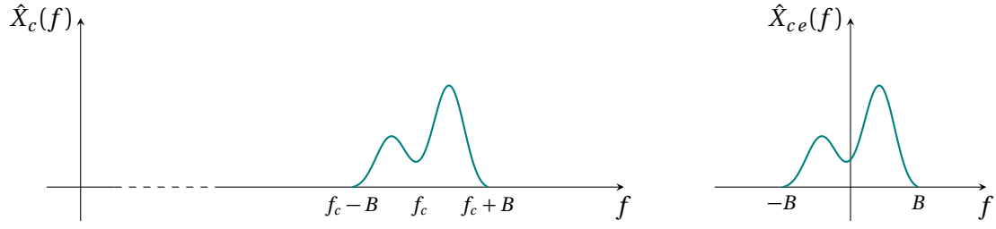
Figura 5.3. Ilustración en frecuencia de la Definición 5.1. La envolvente compleja contiene toda la información del mensaje en la banda alrededor de f_c , llevada a banda base. Como el espectro no es necesariamente simétrico alrededor de f_c , x_{ce} puede ser compleja a pesar de que x_c sea real.
