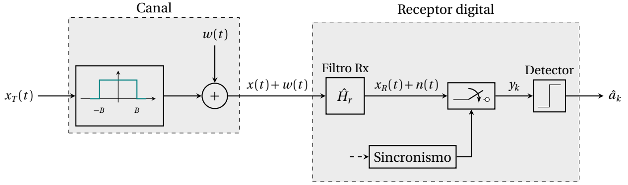
Figura 4.6. Transmisión digital sobre un canal ideal de ancho B con ruido aditivo blanco y Gaussiano.
