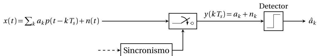
Figura 4.1. Onda PAM afectada por ruido y sistema de detección.
