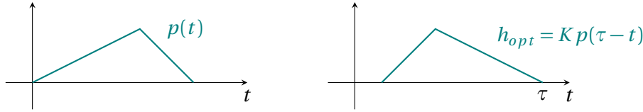
Figura 4.8. Filtro acoplado para un pulso genérico p(t) .
