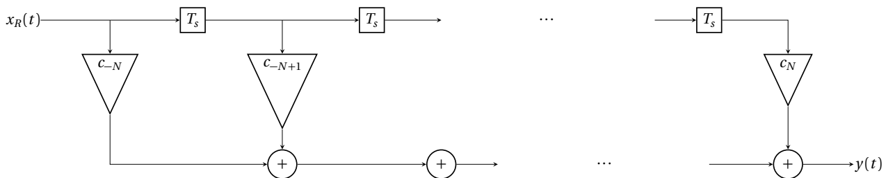
Figura 3.6. Filtro ecualizador
