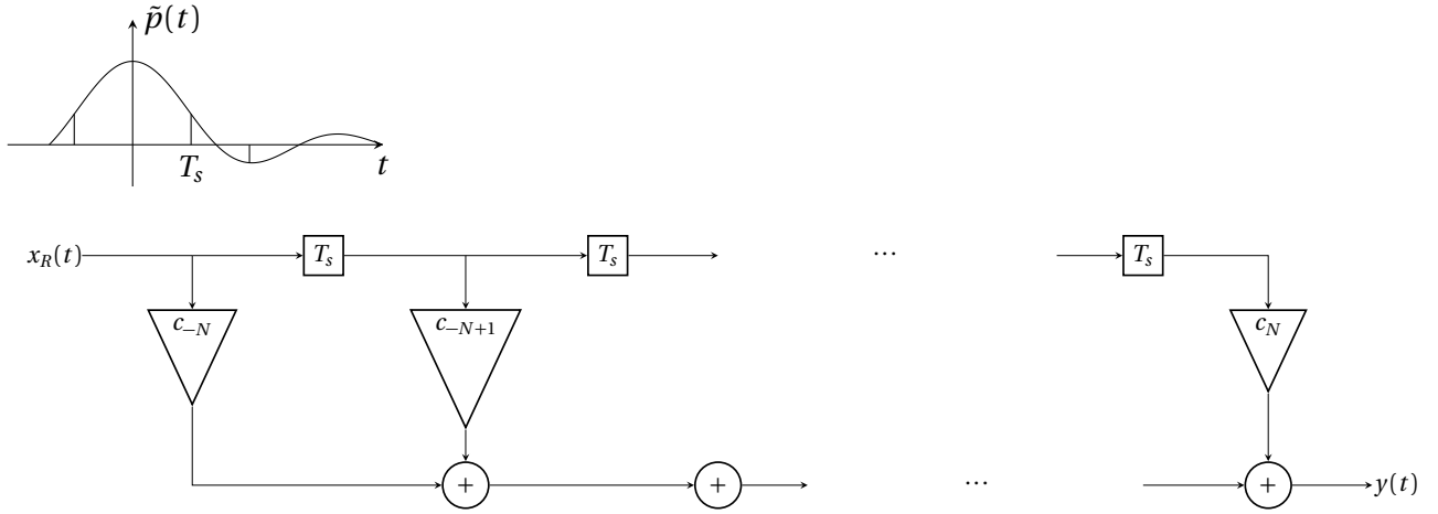
Figura 4.1. Filtro ecualizador
