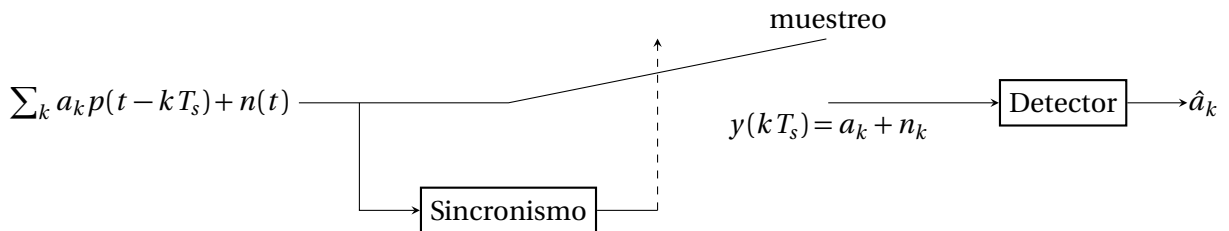
Figura 4.1. Onda PAM afectada por ruido y sistema de detección.
