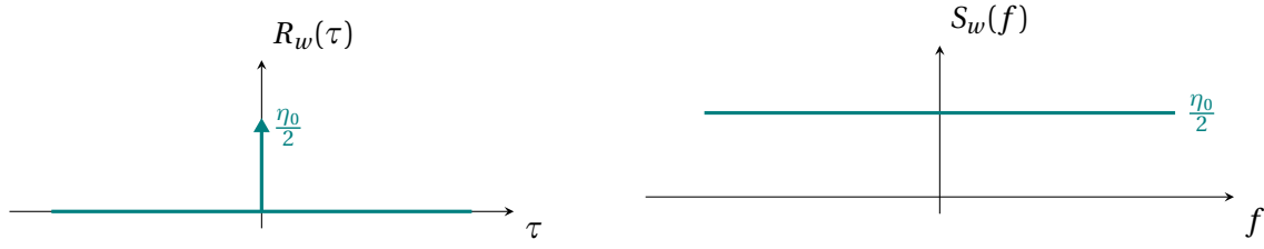
Figura 2.4. Autocorrelación y densidad espectral del ruido blanco gaussiano.
