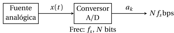
Figura 1.3. Conversión analógica a digital.
