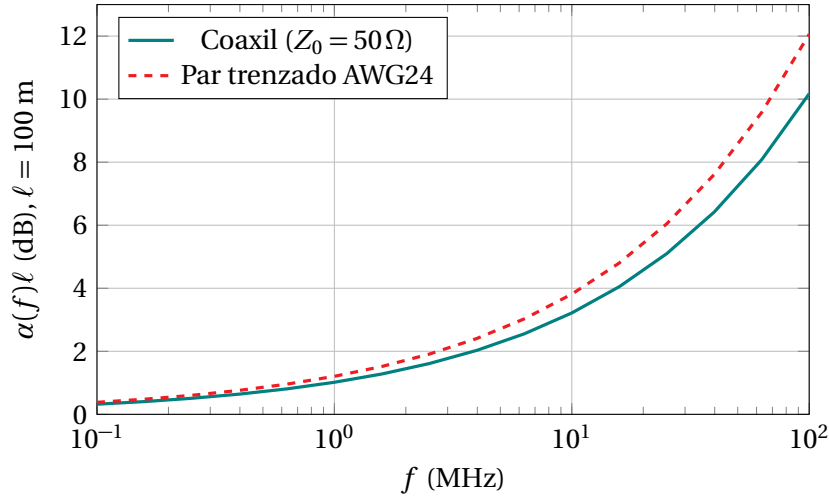
Figura 6.3. Atenuación \alpha(f)\ell en función de la frecuencia, para 100 m de los dos cables del Ejemplo 6.4. La curva crece como \sqrt{f} (efecto pelicular): es la versión física del bloque pasabajos \hat{H}(f) de la Figura 3.7.
