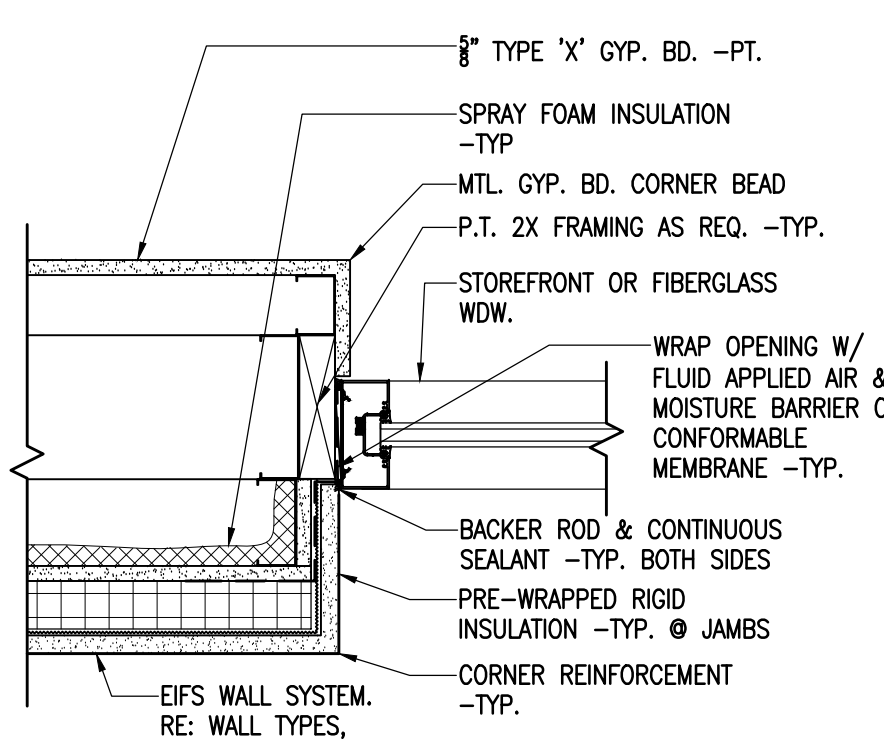
9 JAMB DETAIL SCALE: 1-1/2" = 1'-0"
