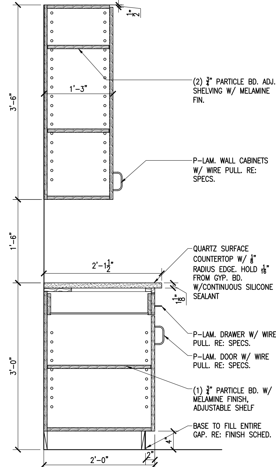
8 CASEWORK DETAIL SCALE: 1"=1'-0"
