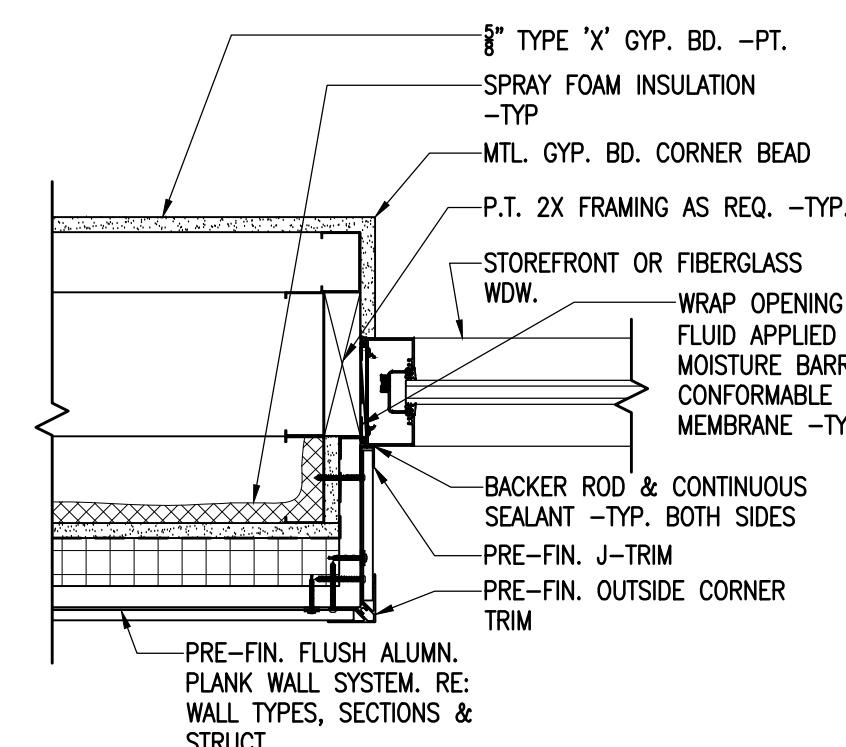
17 JAMB DETAIL SCALE: 1-1/2" = 1'-0"
