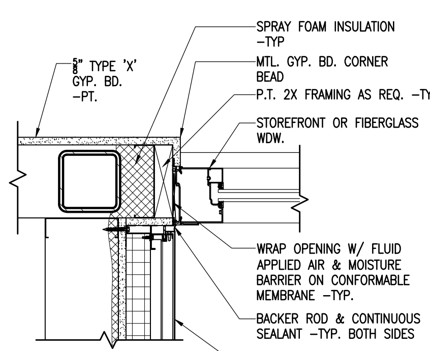
8 JAMB DETAIL SCALE: 1-1/2" = 1'-0"
