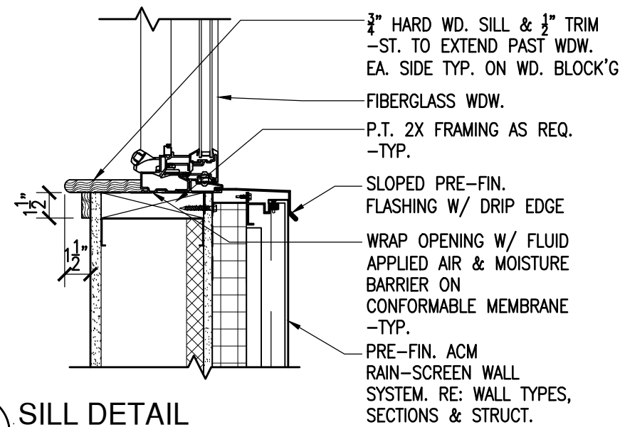
18 SILL DETAIL SCALE: 1-1/2" = 1'-0"
