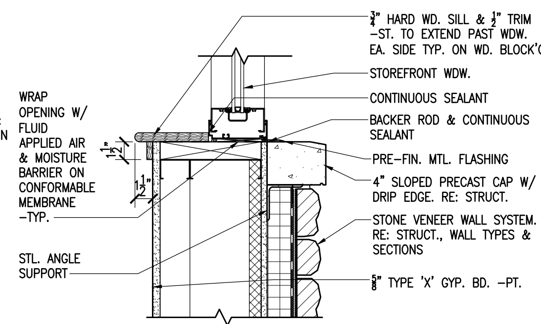
16 SILL DETAIL SCALE: 1-1/2" = 1'-0"
