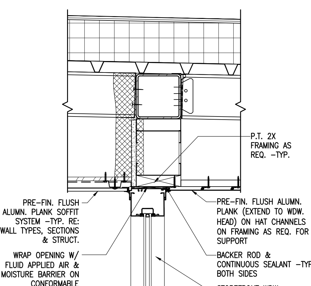
6 HEAD DETAIL SCALE: 1-1/2" = 1'-0"
