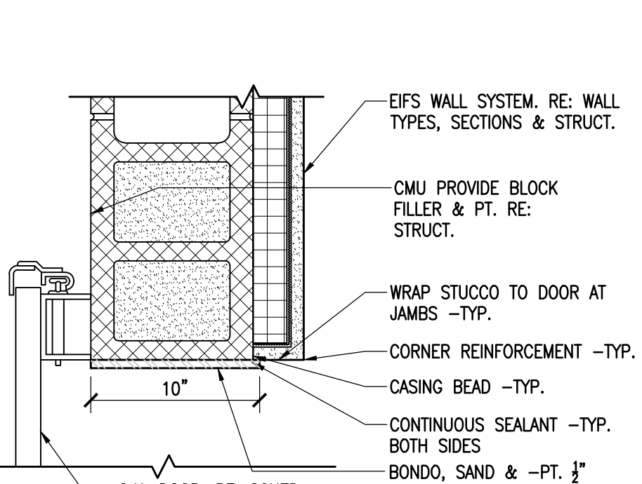
2 JAMB DETAIL SCALE: 1-1/2" = 1'-0"
