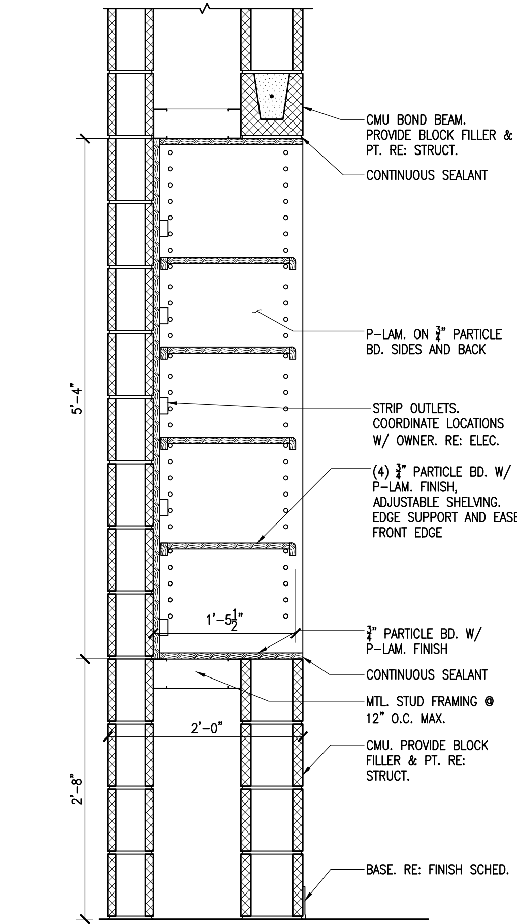
10 CASEWORK DETAIL - APPARATUS BAYS SCALE: 1"=1'-0"
