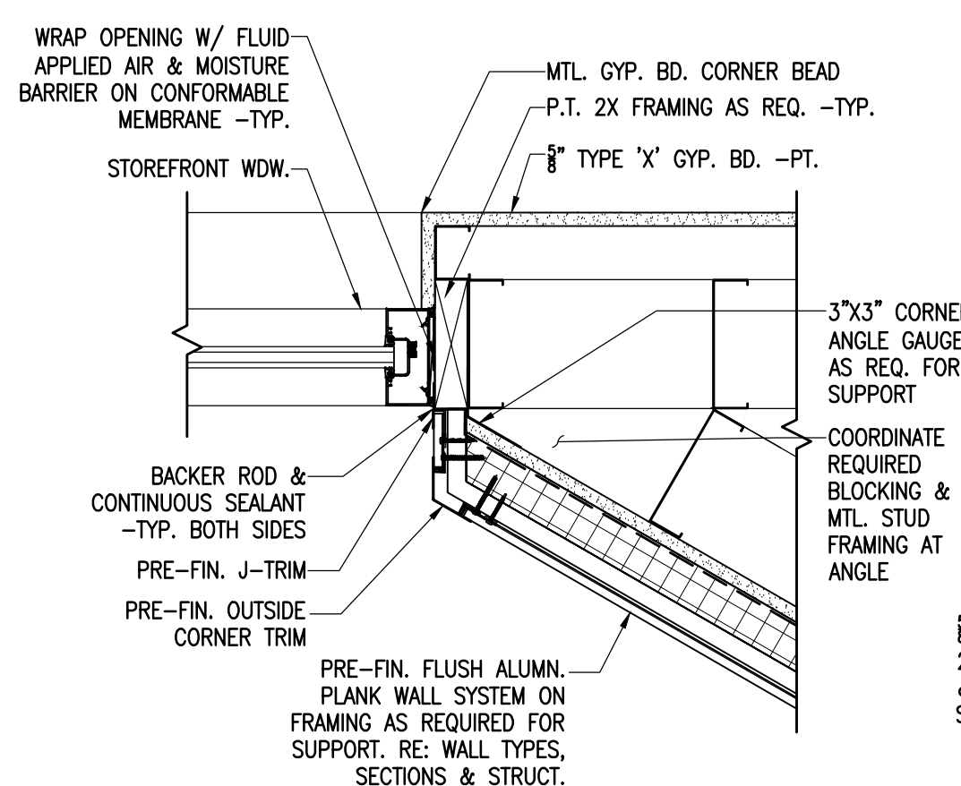
14 JAMB DETAIL SCALE: 1-1/2" = 1'-0"
