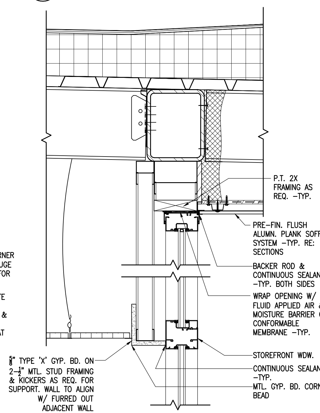
13 HEAD DETAIL SCALE: 1-1/2" = 1'-0"
