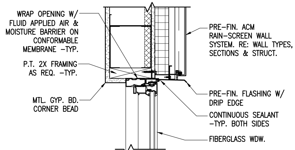
19 HEAD DETAIL SCALE: 1-1/2" = 1'-0"
