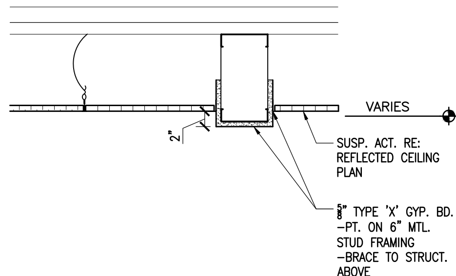
3 HEADER DETAIL SCALE: 1"=1'-0"
