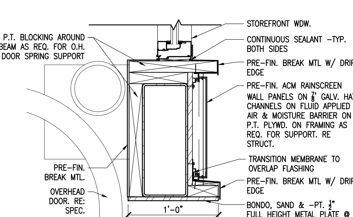
3 HEAD DETAIL SCALE: 1-1/2" = 1'-0"
