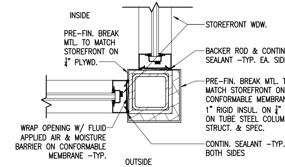
15 JAMB DETAIL SCALE: 1-1/2" = 1'-0"
