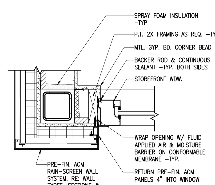
7 JAMB DETAIL SCALE: 1-1/2" = 1'-0"
