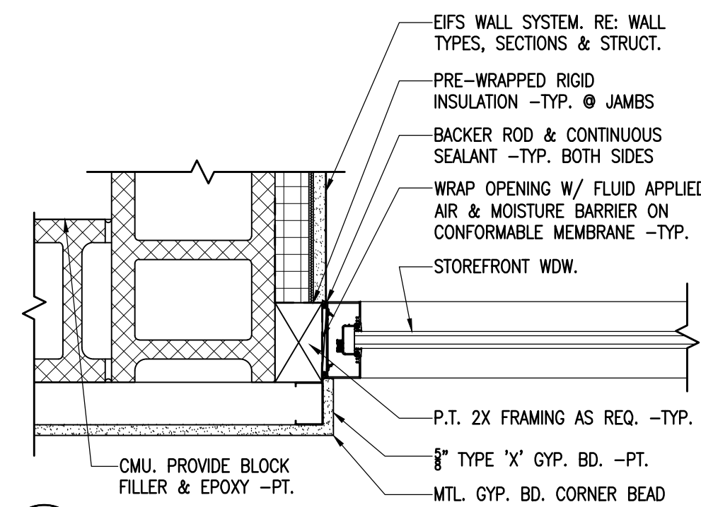
20 JAMB DETAIL SCALE: 1-1/2" = 1'-0"
