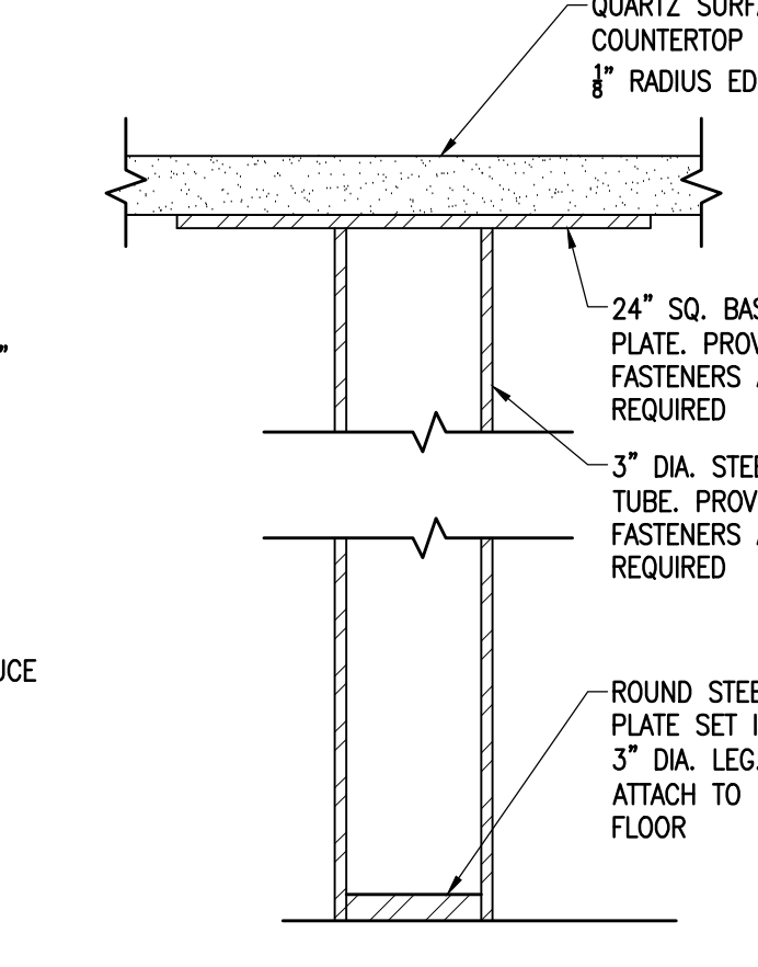
10 DESK LEG DETAIL SCALE: 3"=1'-0"
