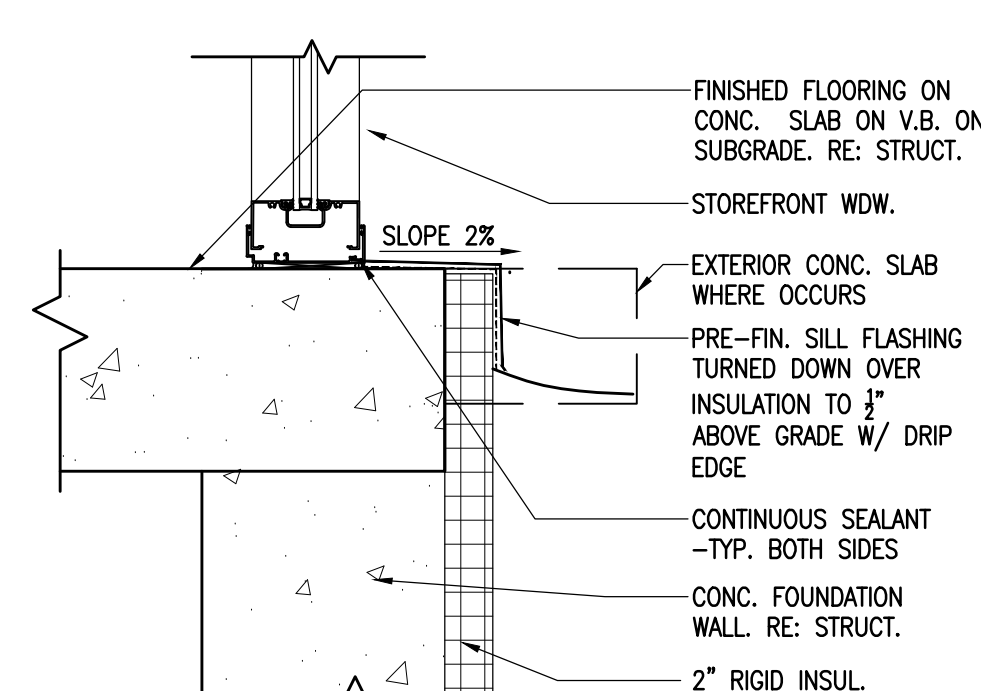
10 SILL DETAIL SCALE: 1-1/2" = 1'-0"
