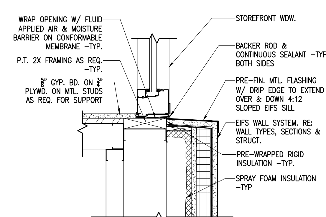
11 SILL DETAIL SCALE: 1-1/2" = 1'-0"
