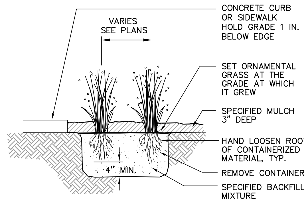
3 ORNAMENTAL GRASS DETAIL N.T.S.
