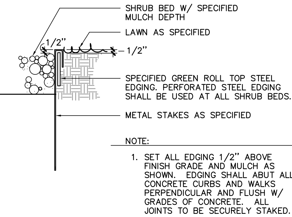
4 STEEL EDGER DETAIL N.T.S.
