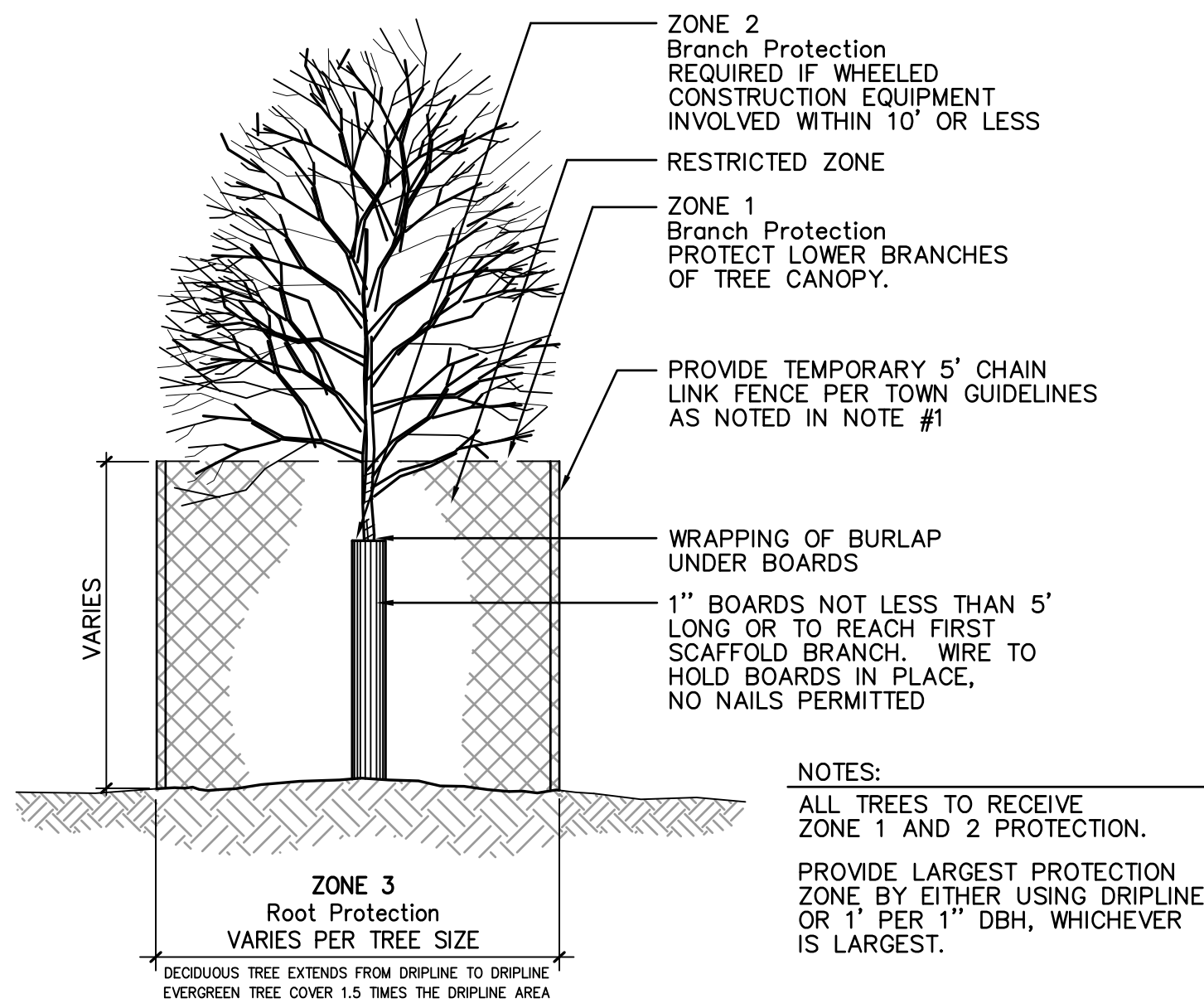
6 EXISTING TREE PROTECTION N.T.S.
