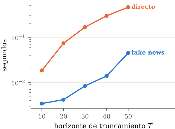
Costo de calcular \mathcal{J}
