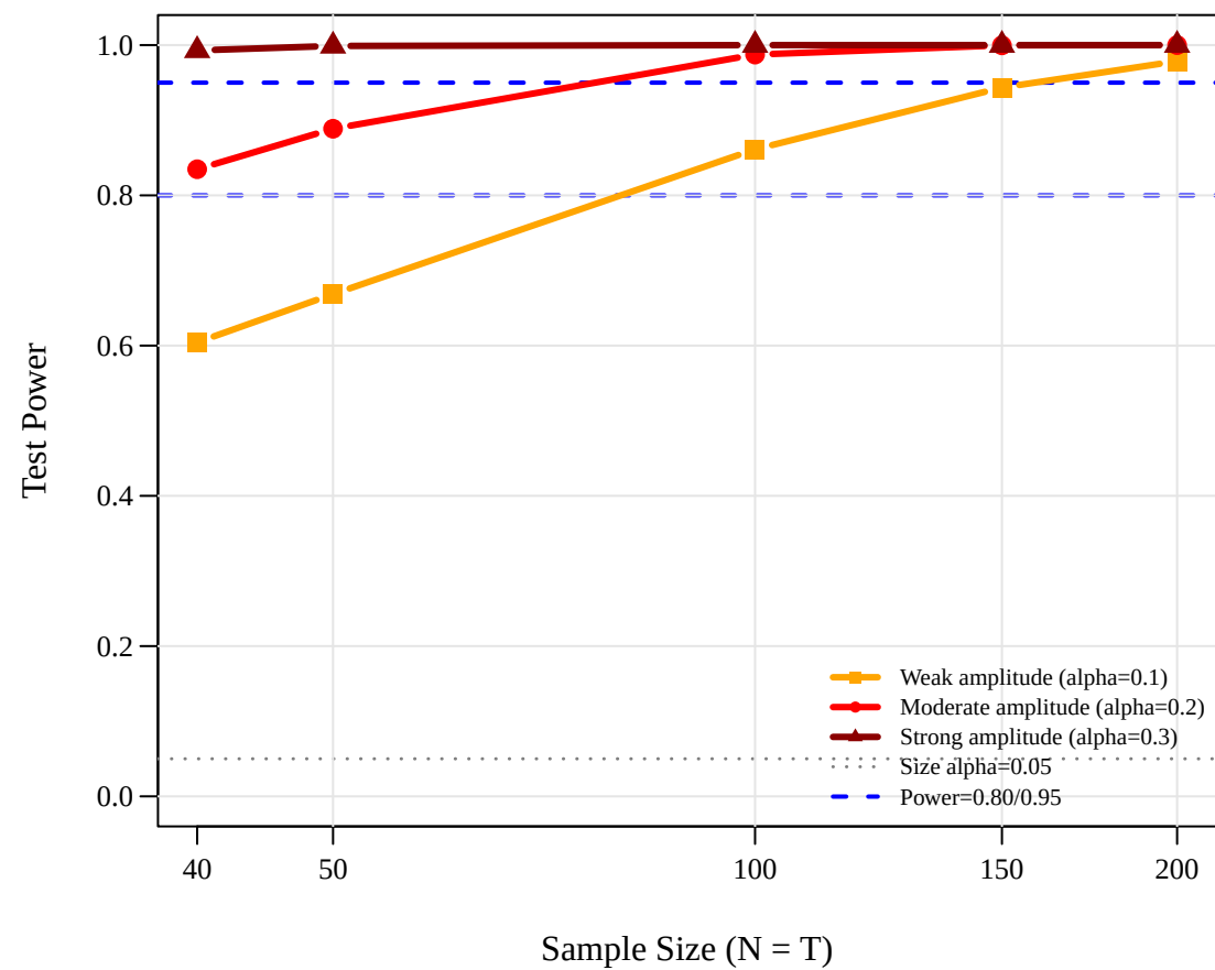
(d) Fourier Test Power (H0: \alpha_1 = \alpha_2 = 0 )
