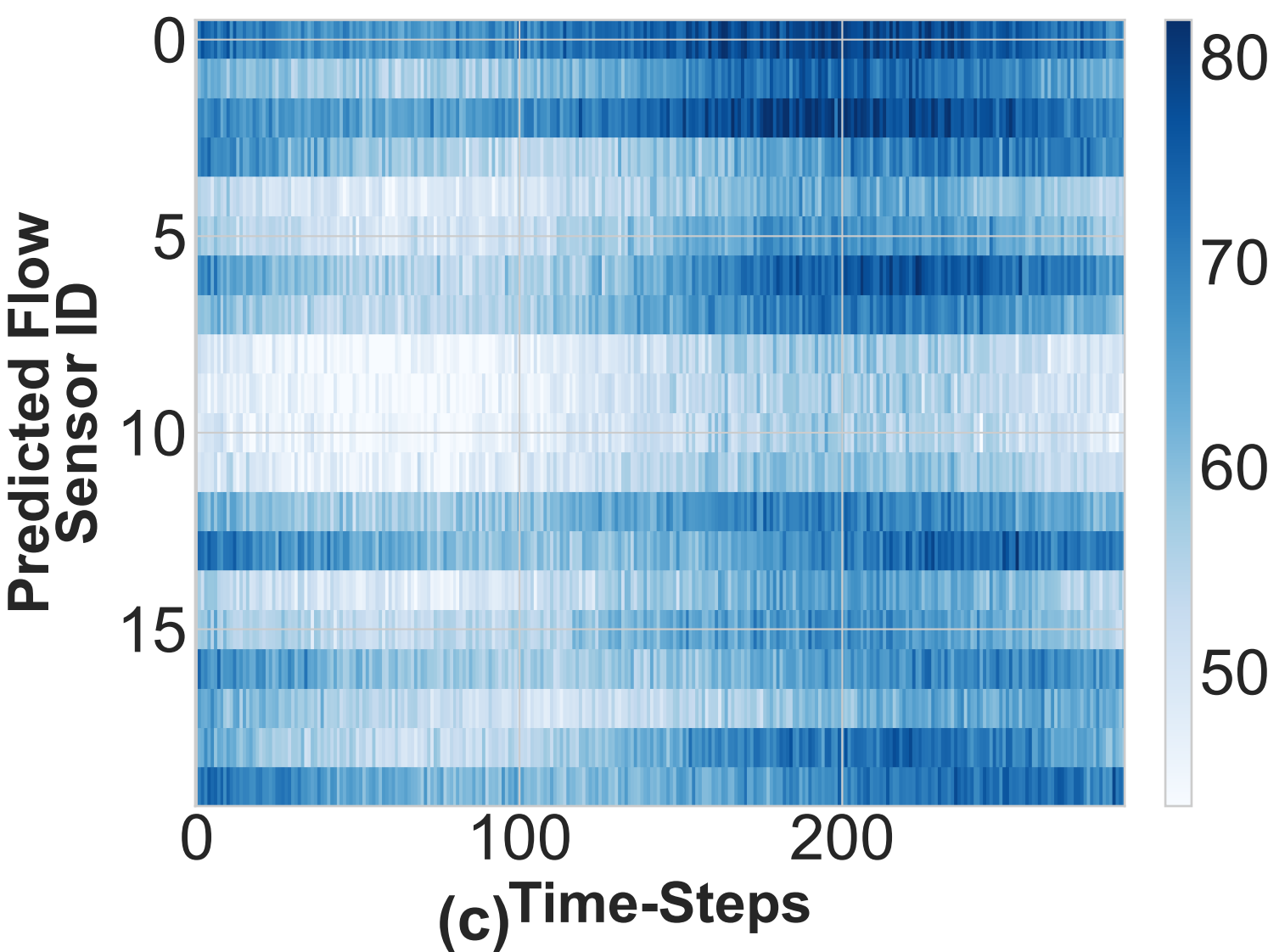
TransGTR Baseline MAE: 1.705
