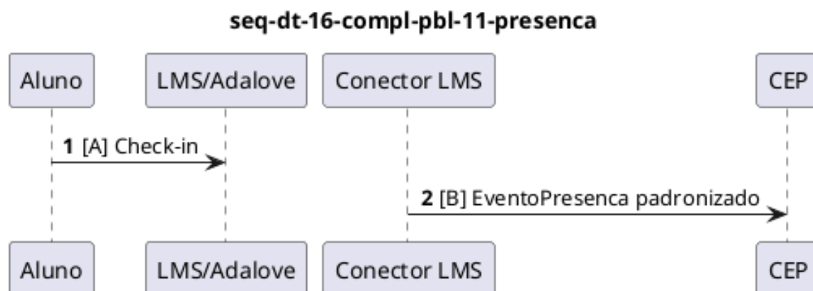
Figura 39: Complemento ao PBL-11 para registro de presença.
