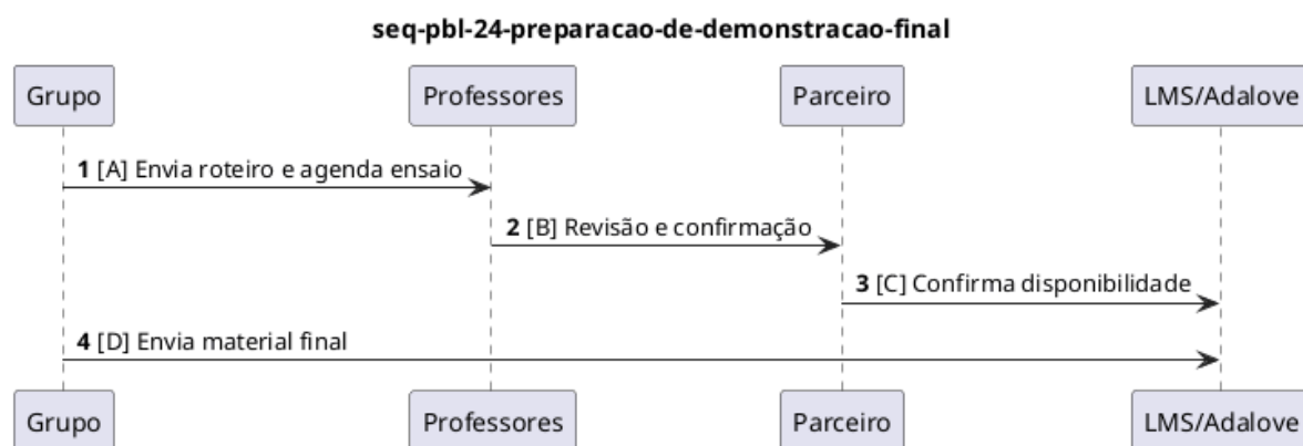
Figura 54: Diagrama de sequência PBL-24 — Preparação de demonstração final.
