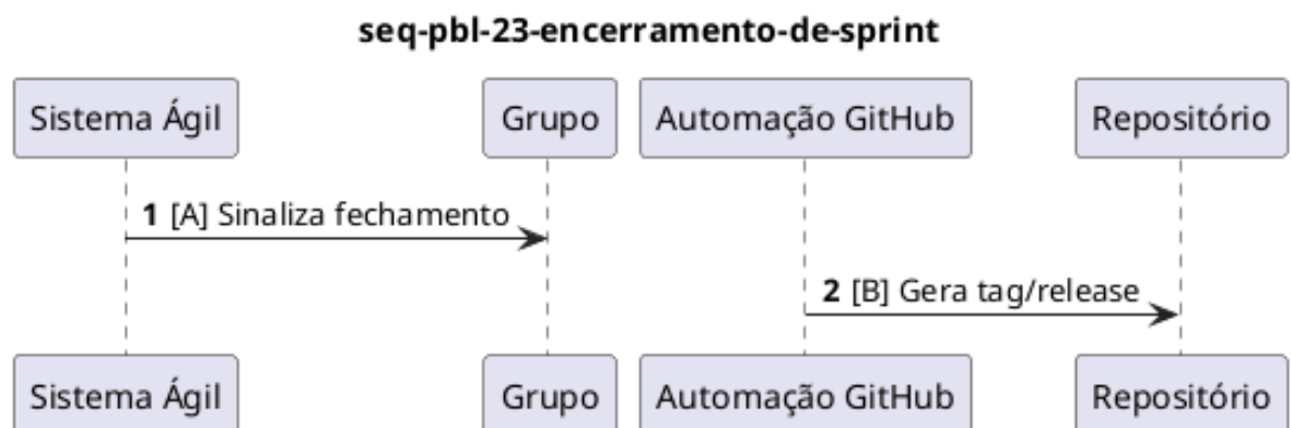
Figura 53: Diagrama de sequência PBL-23 — Encerramento de sprint.
