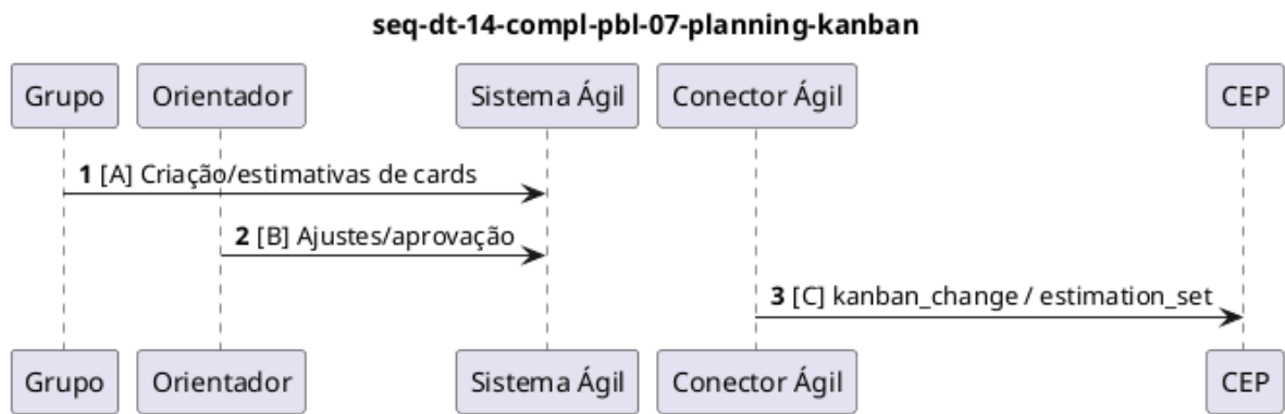
Figura 37: Complemento ao PBL-07 com integração ao Kanban.
