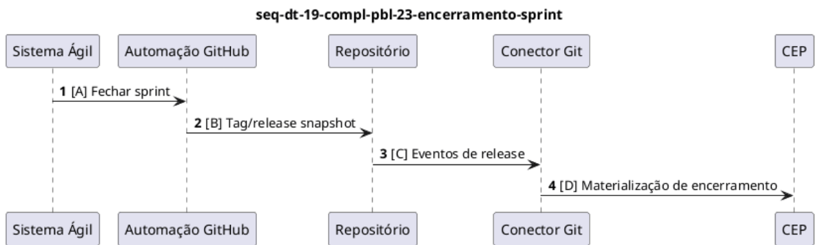
Figura 42: Complemento ao PBL-23 para encerramento de sprint.
