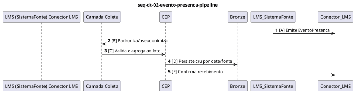
Figura 13: Pipeline do evento de presença: captura, validação, enriquecimento e persistência.
