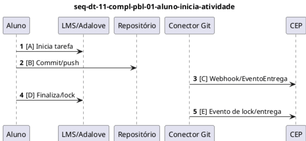
Figura 34: Complemento ao PBL-01 na visão do gêmeo digital.
