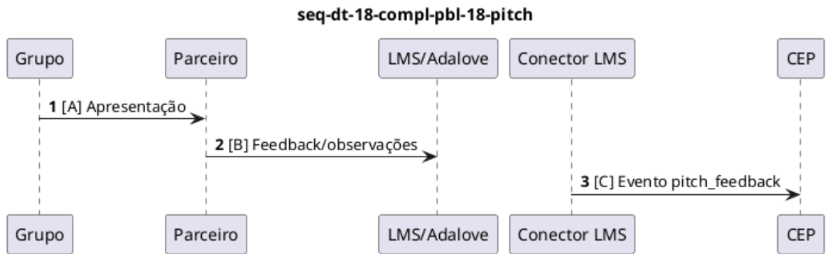
Figura 41: Complemento ao PBL-18 para pitch.
