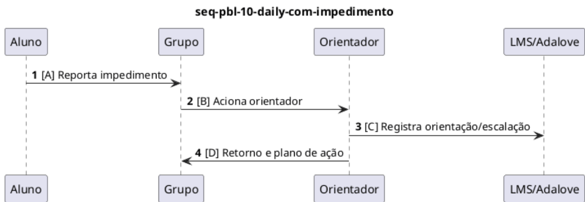
Figura 23: Diagrama de sequência PBL-10 — Daily com impedimento.
