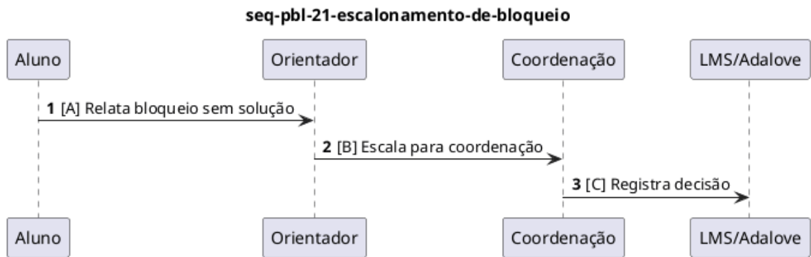
Figura 51: Diagrama de sequência PBL-21 — Escalonamento de bloqueio.
