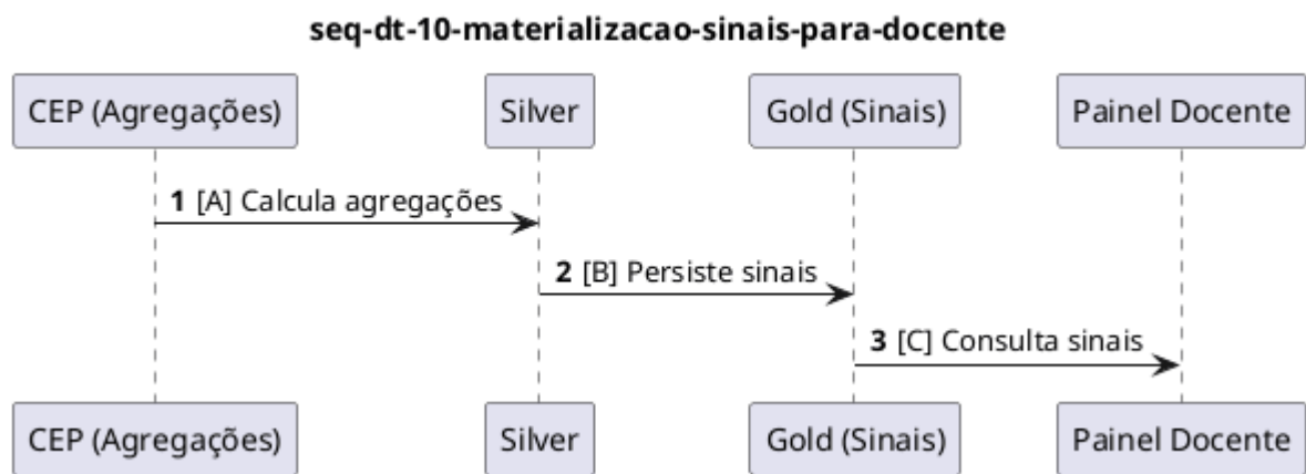
Figura 33: Materialização de sinais e dashboards para docentes.
