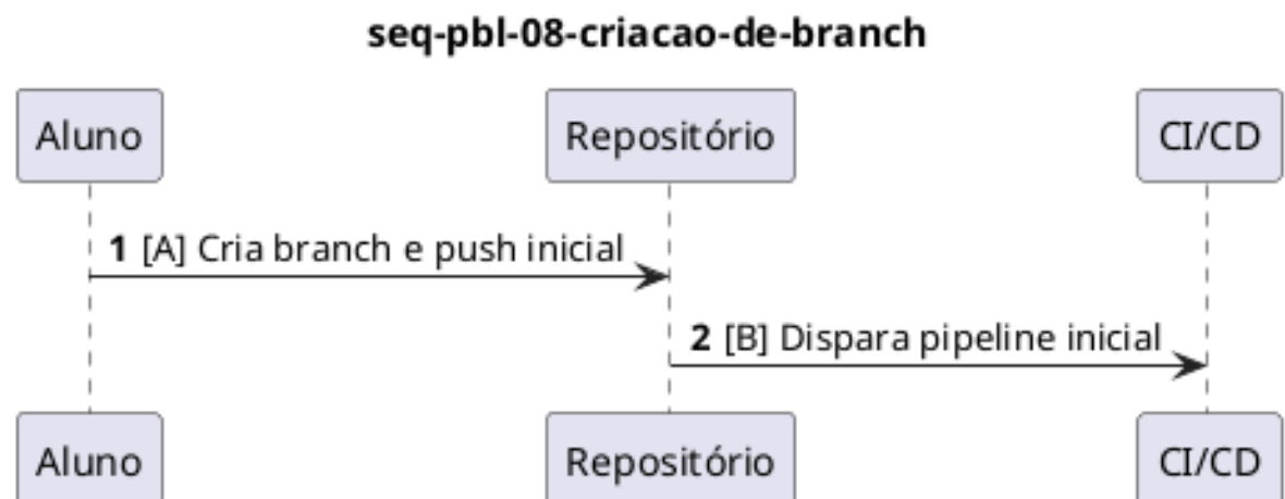
Figura 21: Diagrama de sequência PBL-08 — Criação de branch.
