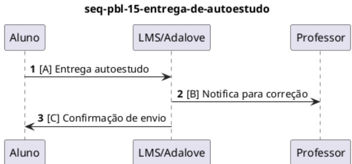
Figura 27: Diagrama de sequência PBL-15 — Entrega de autoestudo.
