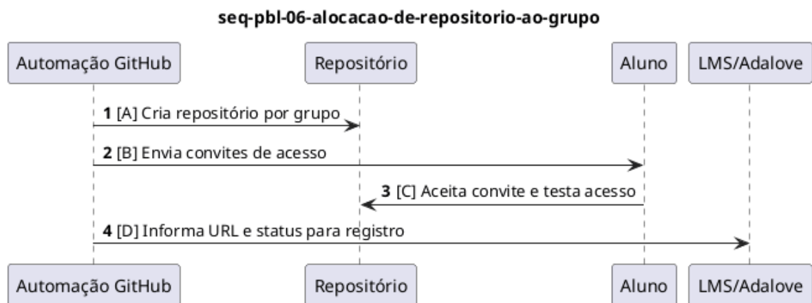
Figura 20: Diagrama de sequência PBL-06 — Alocação de repositório ao grupo.
