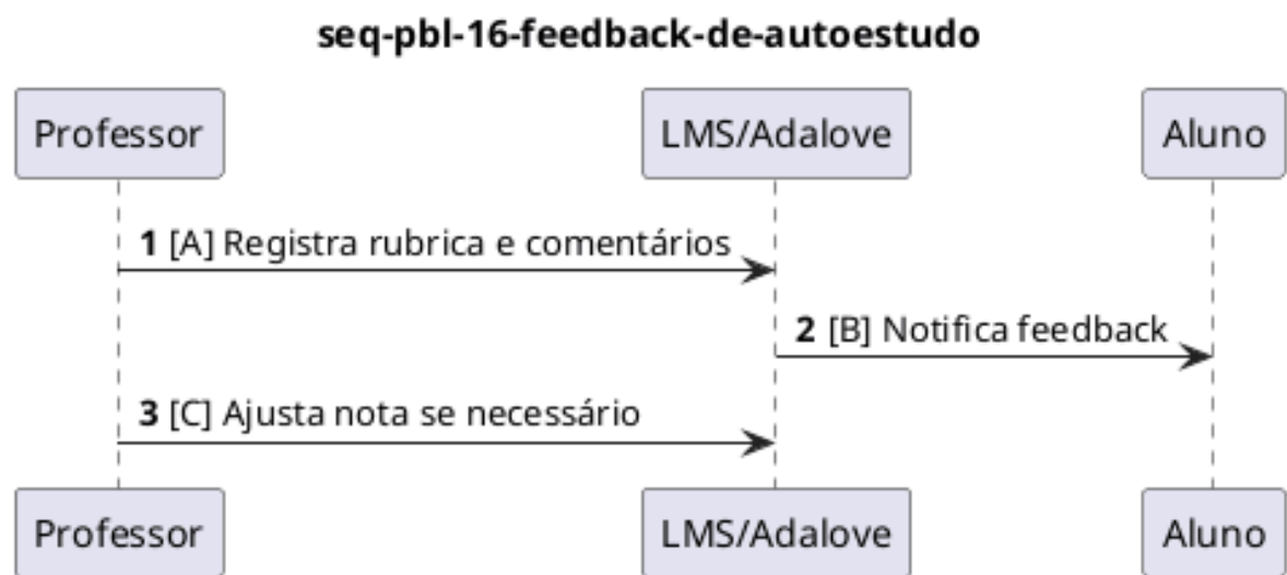
Figura 46: Diagrama de sequência PBL-16 — Feedback de autoestudo.
