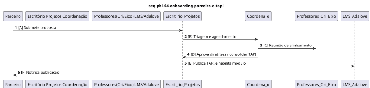
Figura 18: Diagrama de sequência PBL-04 — Onboarding do parceiro e TAPI.
