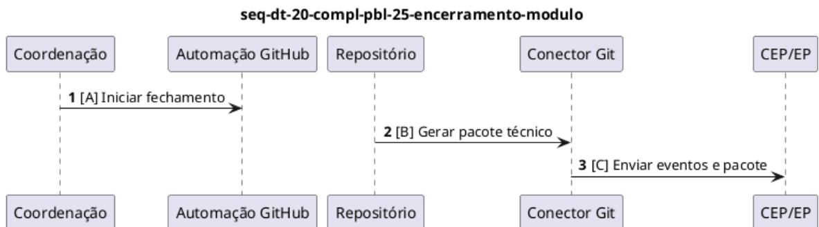
Figura 43: Complemento ao PBL-25 para encerramento de módulo.
