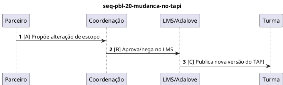
Figura 50: Diagrama de sequência PBL-20 — Mudança no TAPI.
