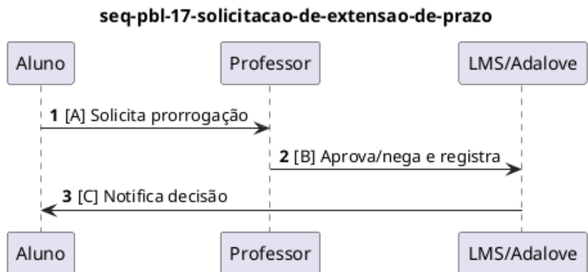
Figura 47: Diagrama de sequência PBL-17 — Solicitação de extensão de prazo.
