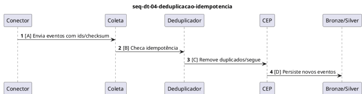
Figura 15: Deduplicação e idempotência na ingestão para evitar eventos repetidos.
