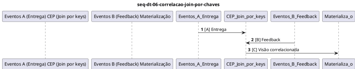
Figura 29: Correlação de eventos via join por chaves canônicas.
