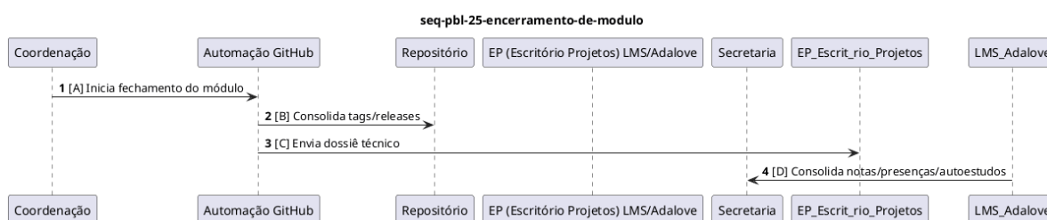
Figura 55: Diagrama de sequência PBL-25 — Encerramento de módulo.
