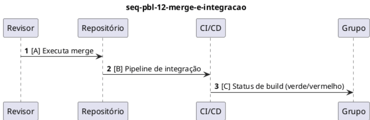
Figura 25: Diagrama de sequência PBL-12 — Merge e integração.
