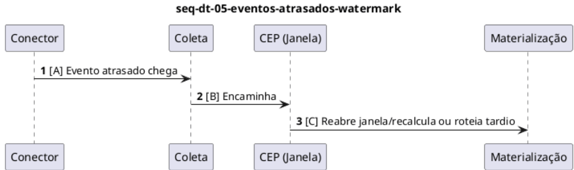
Figura 28: Eventos atrasados: tratamento com watermark temporal.
