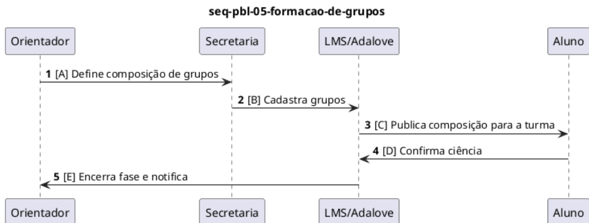
Figura 19: Diagrama de sequência PBL-05 — Formação de grupos.
