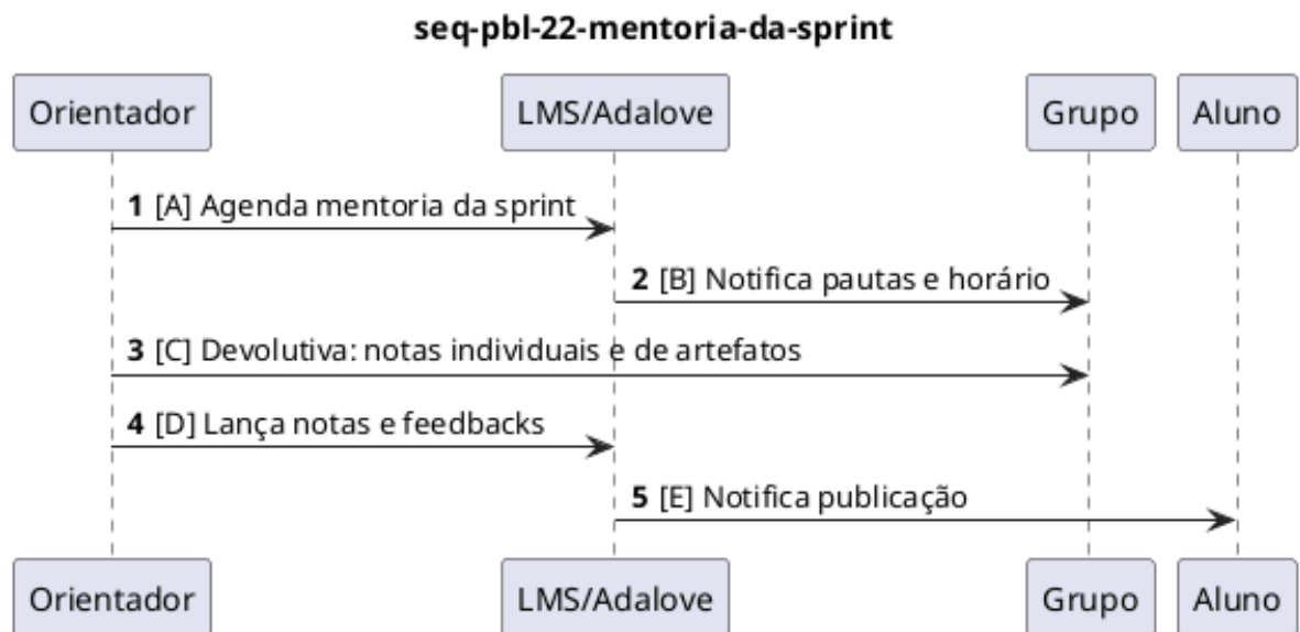
Figura 52: Diagrama de sequência PBL-22 — Mentoria da sprint.
