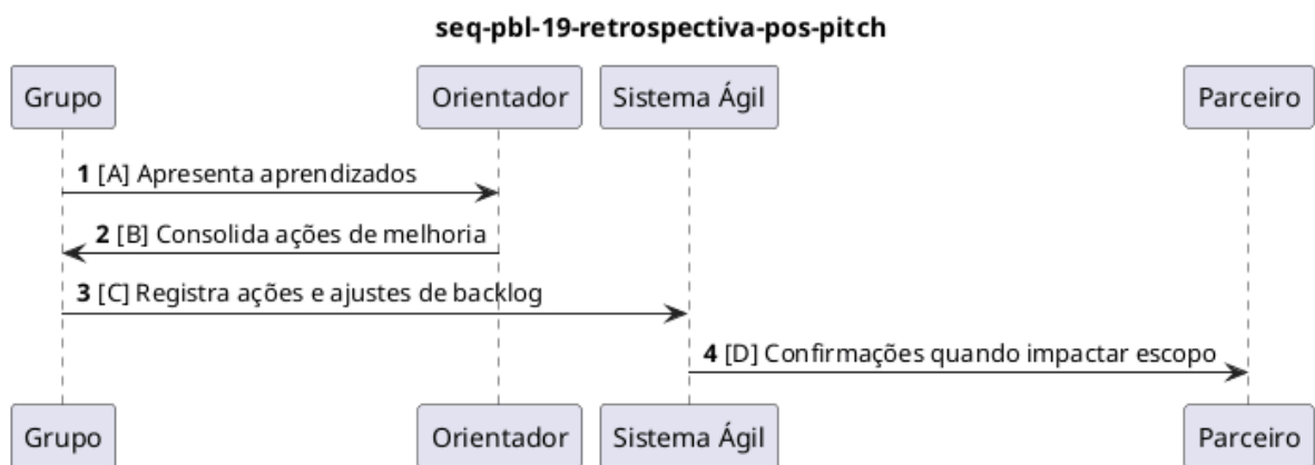
Figura 49: Diagrama de sequência PBL-19 — Retrospectiva pós-pitch.
