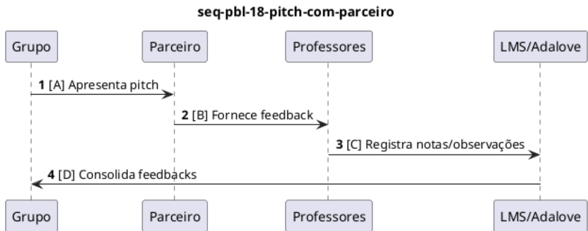
Figura 48: Diagrama de sequência PBL-18 — Pitch com parceiro.
