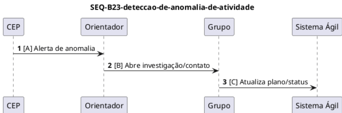
Figura 45: Detecção de anomalias de atividade a partir de métricas de eventos.
