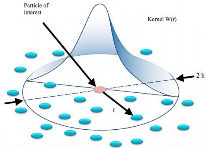
Figura 3.3. Representación visual de la función de kernel W(r, h) sobre un sistema de partículas. El parámetro h define el límite del soporte compacto, fuera del cual las interacciones entre partículas se asumen nulas.
