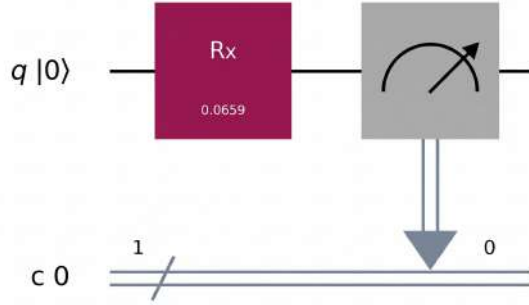
Figura 5.1. Implementación de un único bloque de Trotter correspondiente a un paso de tiempo \Delta t = 0,3 . La interacción del kernel SPH se traduce en una rotación R_x sobre los qubits del sistema.
