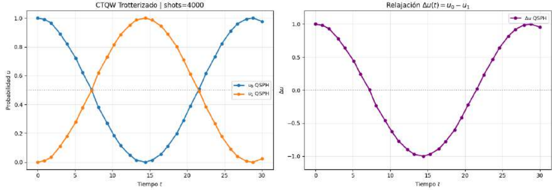
Figura 5.2. Evolución temporal de las poblaciones P_j en el circuito unitario (CTQW cerrado).
