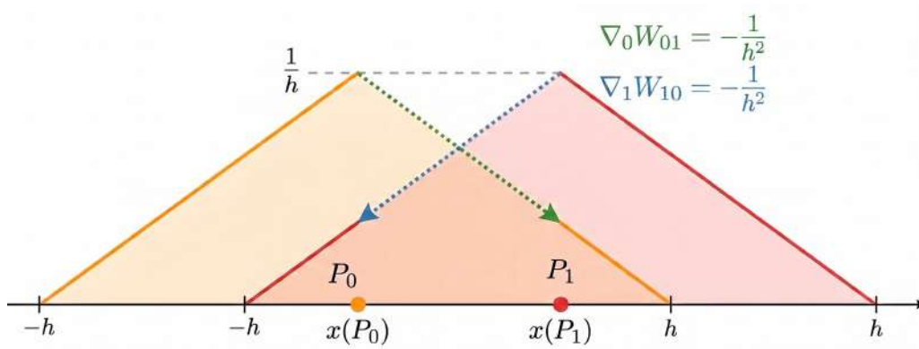
Figura 4.1. Esquema geométrico del kernel triangular y la dirección de interacción entre partículas.
