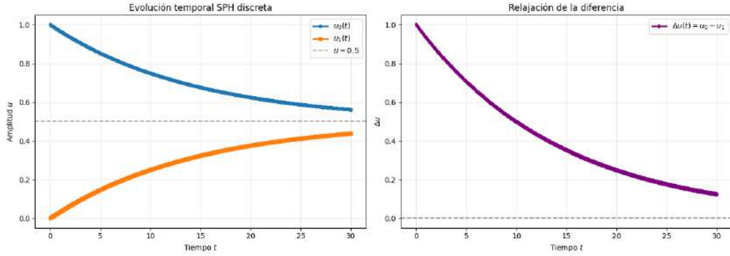
Figura 6.5. Simulación clásica con c = 10^{-1} .
