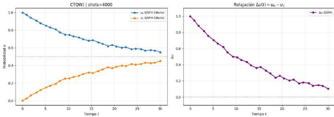
Figura 6.6. Simulación cuántica con c = 10^{-1} .
