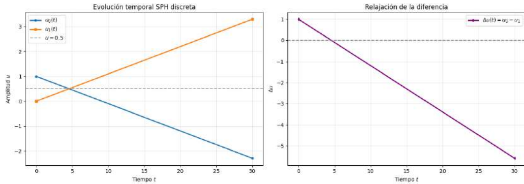
Figura 6.4. Lectura directa del estado inicial y del estado a t = 30 con simulación clásica
