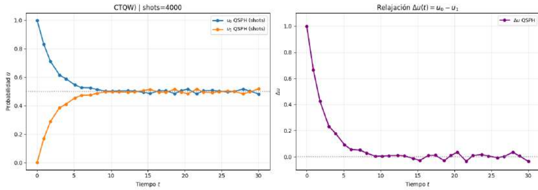
Figura 6.8. Simulación cuántica con c = 10^{-0,2} .
