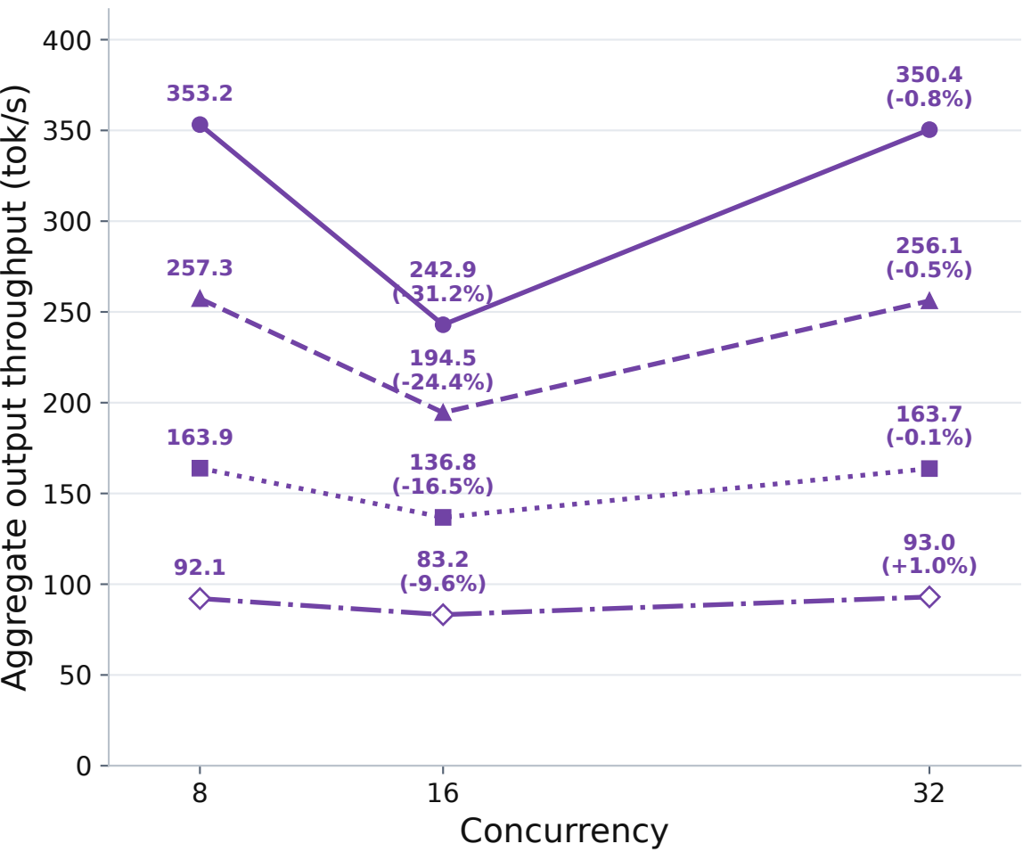
IQ1_M
