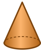
مخروط
