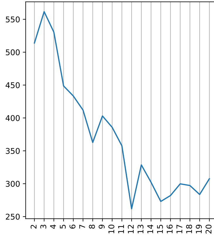
Harabasz score
