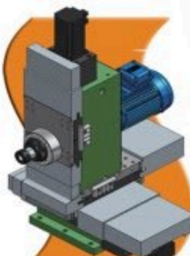
三軸伺服磨銼主軸頭 Spindle with XYZ Slide
