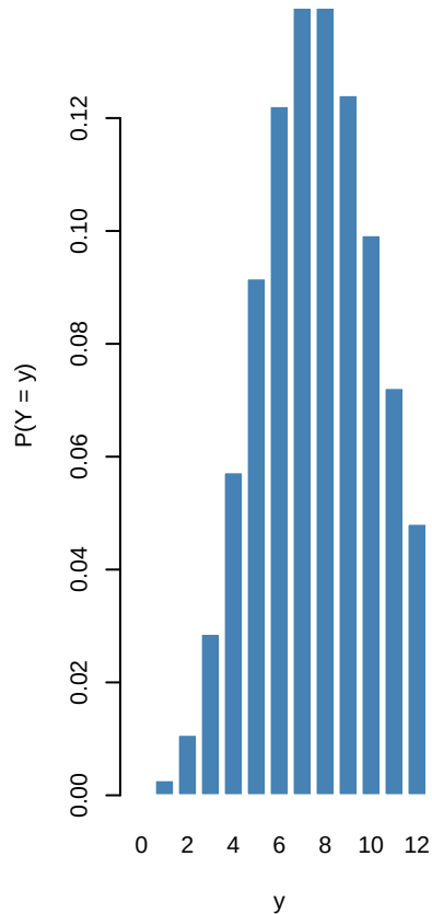
Poisson(8)
