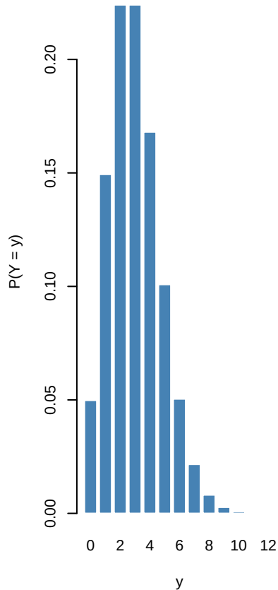
Poisson(3)
