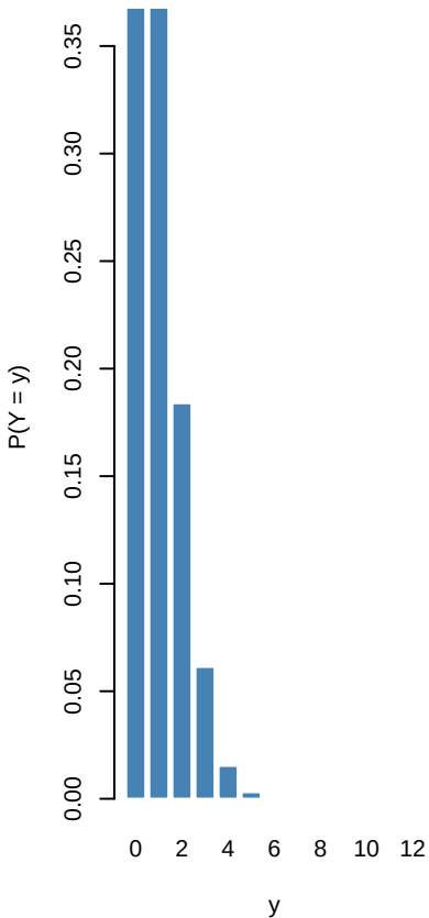
Poisson(1)
