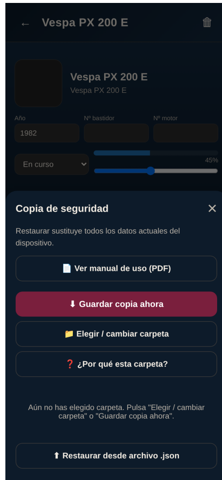
Panel de copia de seguridad, accesible desde el icono de flechas de la pantalla principal.
