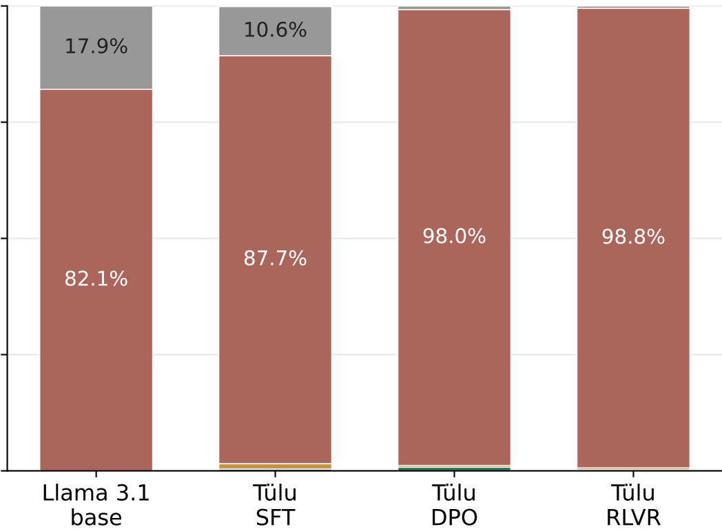
Llama 3.1-Tulu 3 70B
