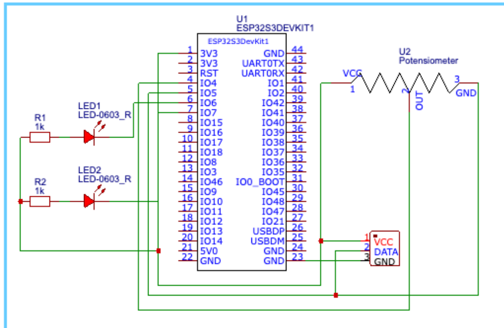
Gambar 12. Skematik Rangkaian Elektronik Trainer Kit
