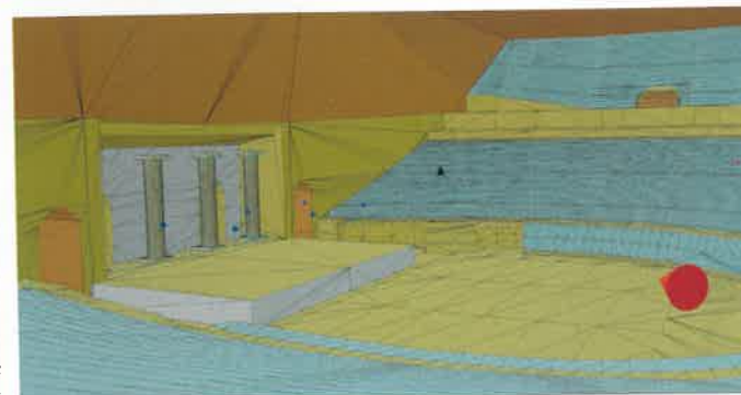
Simulation acoustique dans le modèle 3D. On définit des sources (en bleu) et des récepteurs (en rouge).
