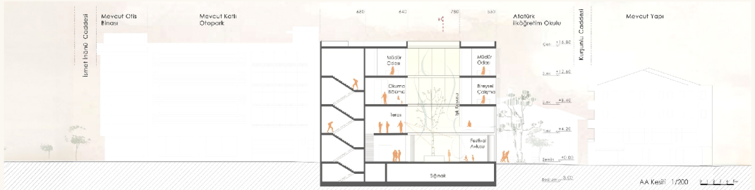
11 AA kesiti — avludan sahneye kamusal zemin; ışık kuyusu üst katları deler.
