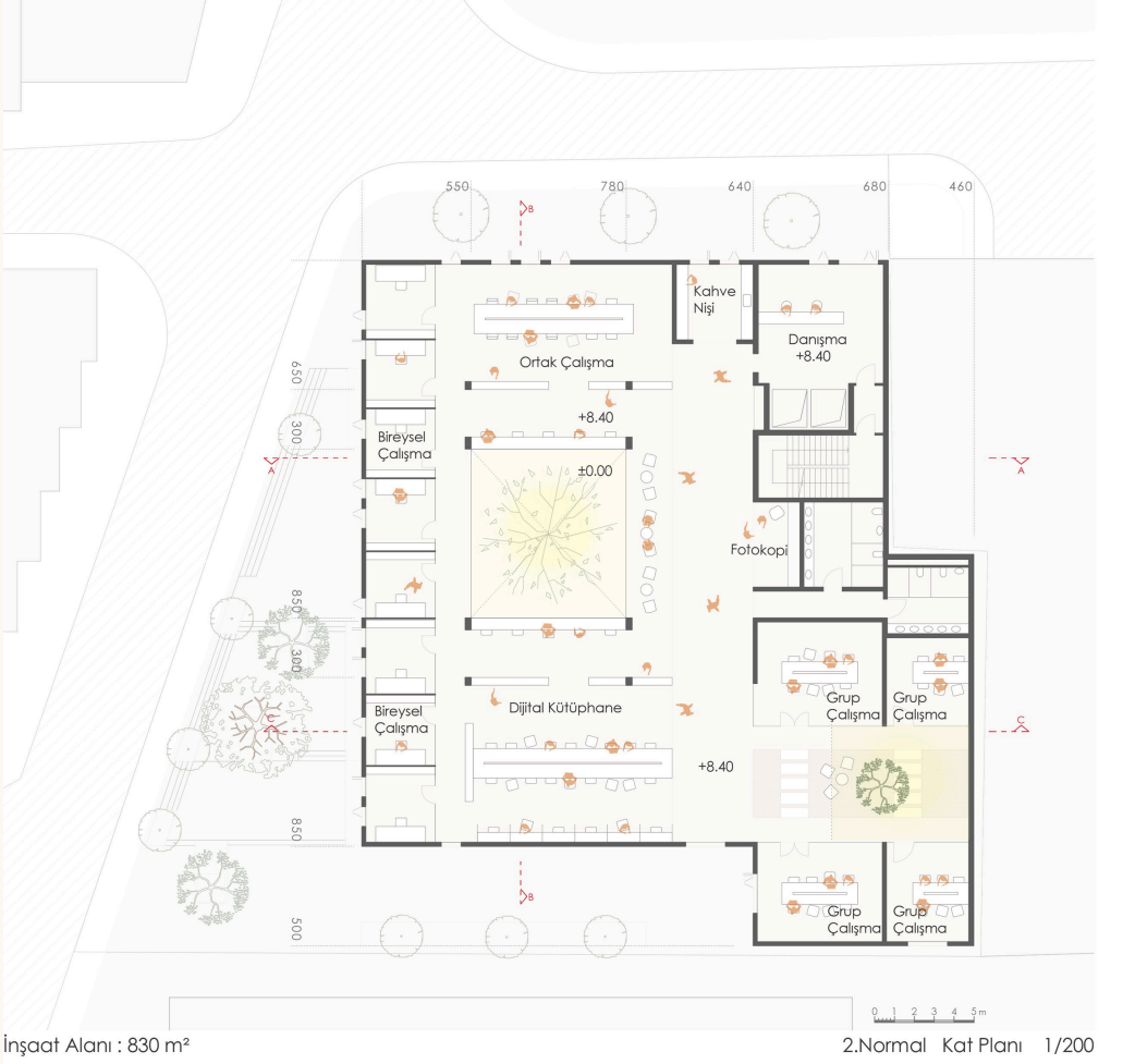
16 İkinci kat planı — ışıık kuyusu çevresinde ortak çalışma; iç bahçe çekirdeğinde grup odaları.
