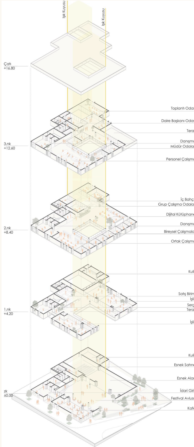
06 Katların açılımı — Işık kuyusu zeminden çatıya tüm katları deler.
