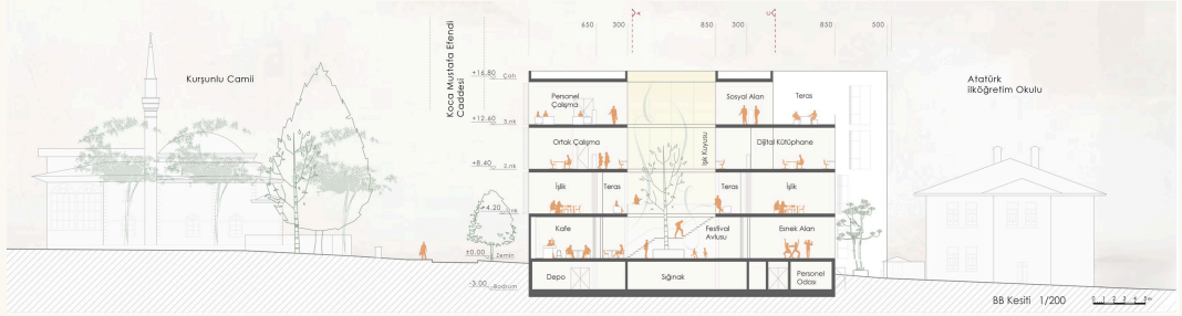
15 BB kesiti — sessiz çalışma kuşağı, ışık kuyusuyla zemindeki kamusal hayata bağlanır.
