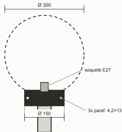
DETALHE — BOCA & GLOBO globo PVC 15×30 incluso · lâmpada não inclusa
