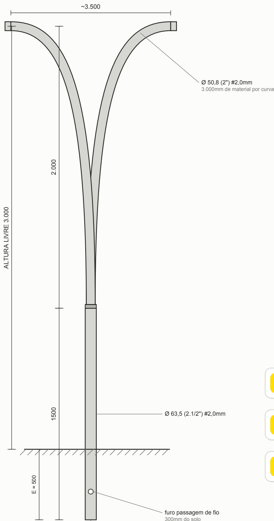
VISTA LATERAL — ENGASTADO
