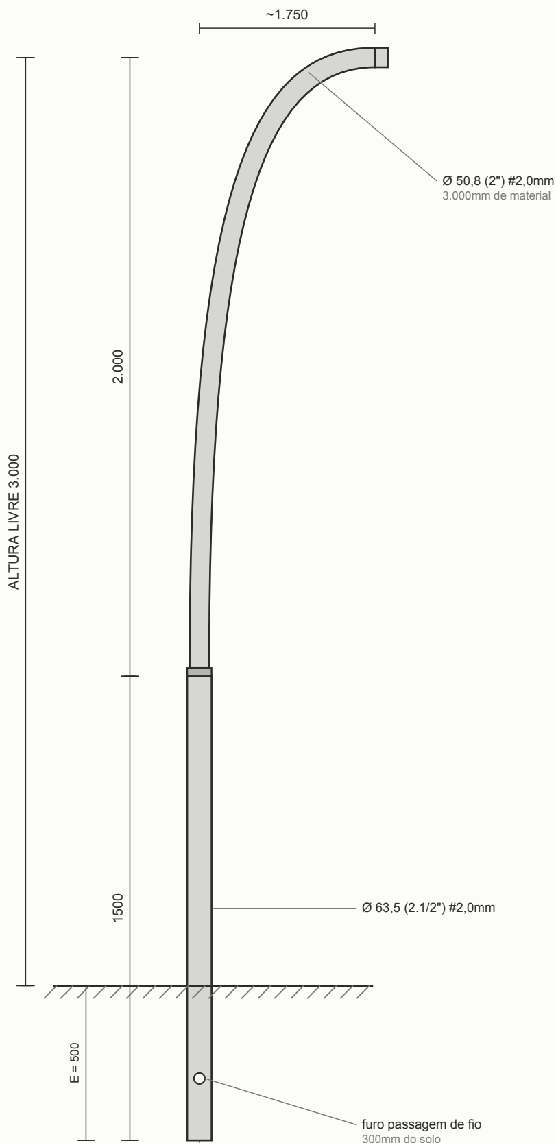
VISTA LATERAL — ENGASTADO
