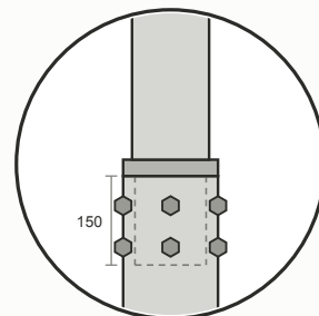
EMENDA MÓVEL encaixe de 150mm com luva interna 6 parafusos sextavados — espaçamento 120°
