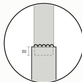
EMENDA FIXA encaixe de 50mm soldado solda circunferencial estrutural
