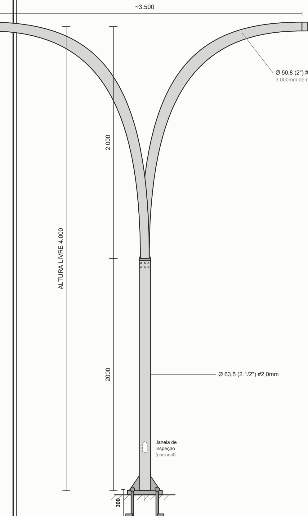
VISTA LATERAL — FLANGEADO medidas em mm
