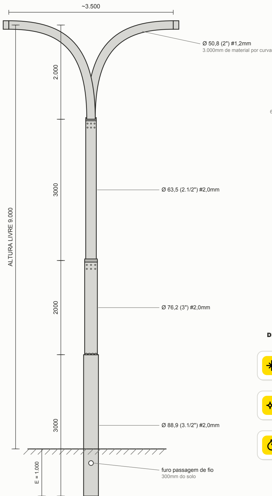
VISTA LATERAL — ENGASTADO
