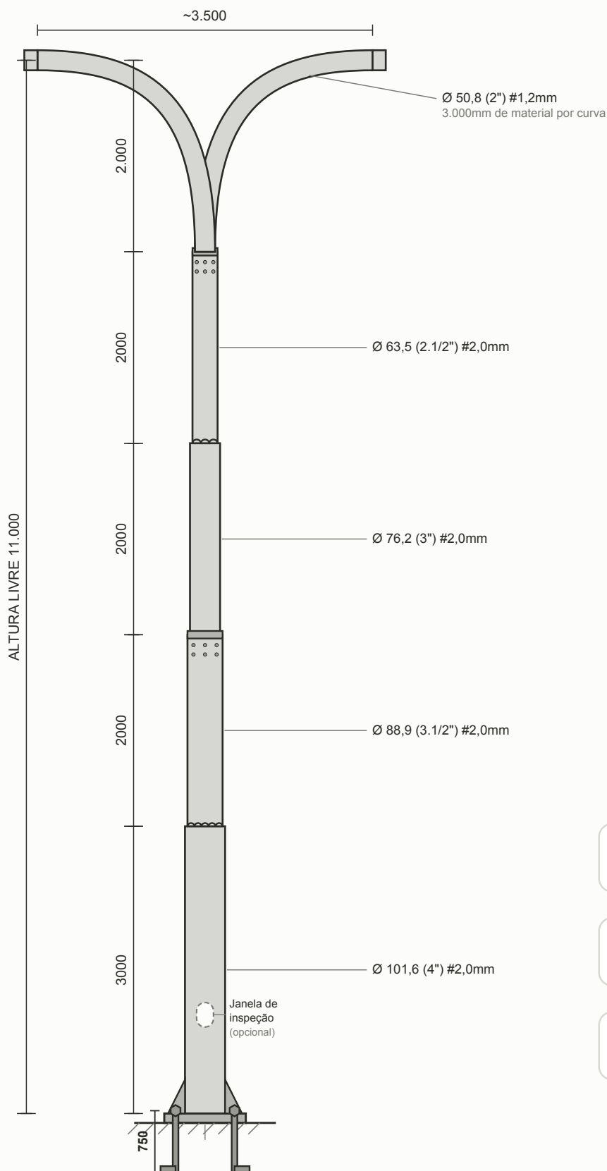
VISTA LATERAL — FLANGEADO medidas em mm
