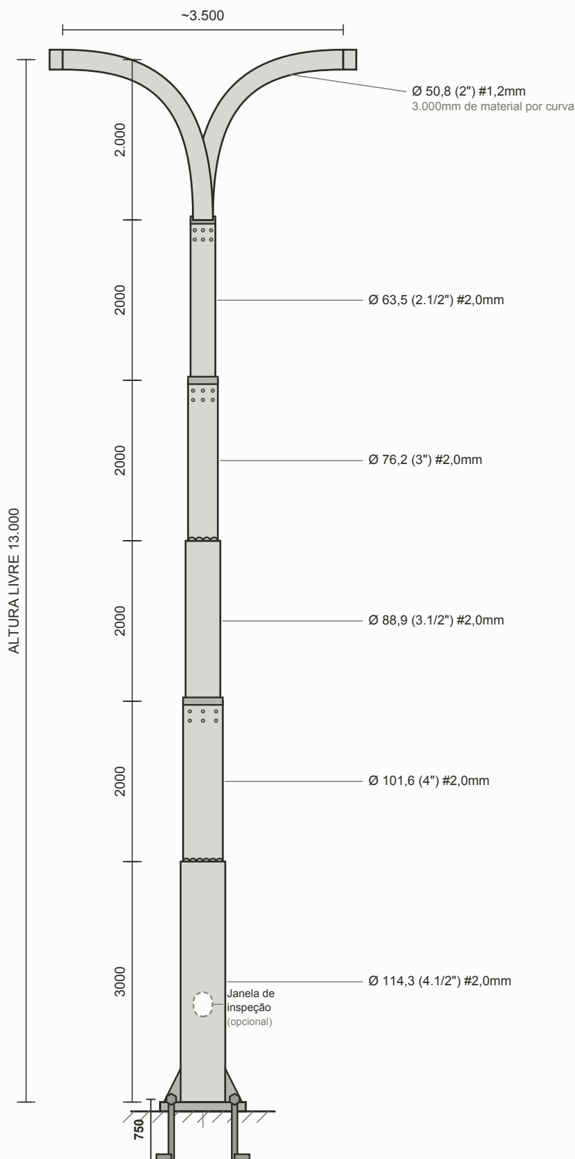
VISTA LATERAL — FLANGEADO medidas em mm
