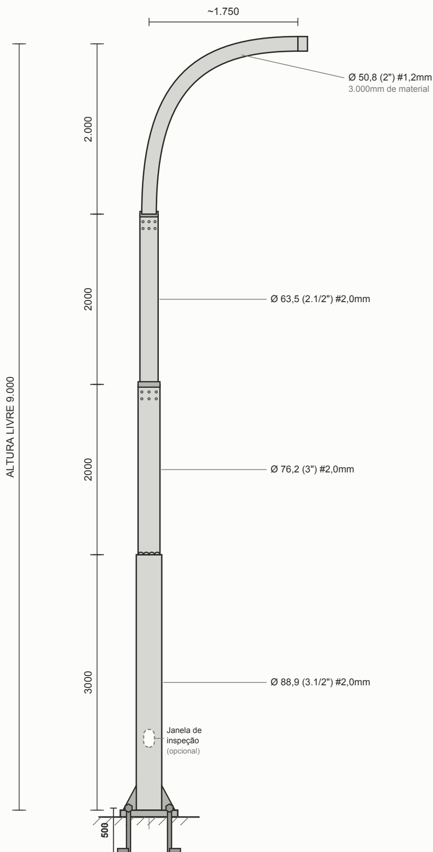
VISTA LATERAL — FLANGEADO medidas em mm
