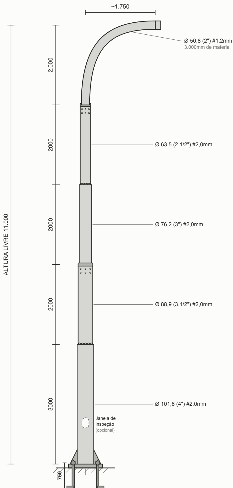
VISTA LATERAL — FLANGEADO medidas em mm
