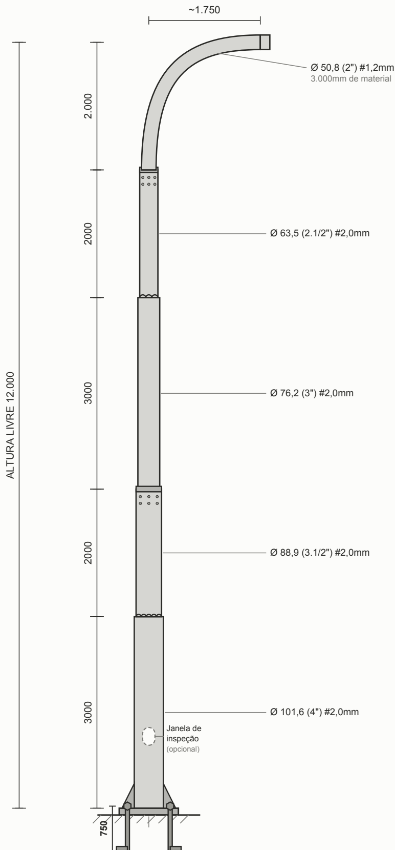
VISTA LATERAL — FLANGEADO medidas em mm
