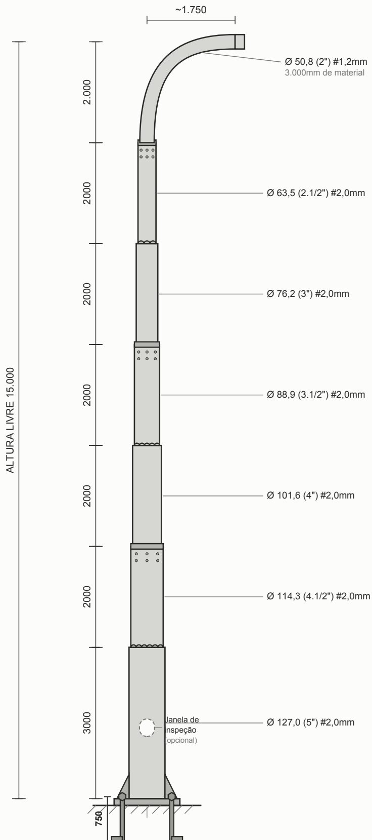
VISTA LATERAL — FLANGEADO medidas em mm
