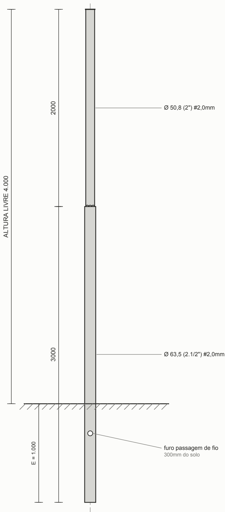
VISTA LATERAL — ENGASTADO
