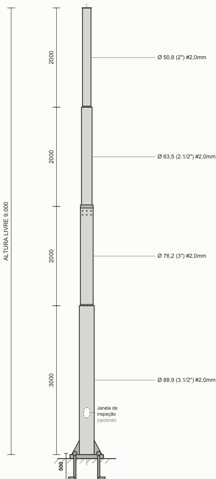
VISTA LATERAL — FLANGEADO medidas em mm
