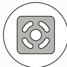
SAPATA / FLANGE placa 330×330mm · chapa 1/2" furos oblongos em curva — nivelamento
