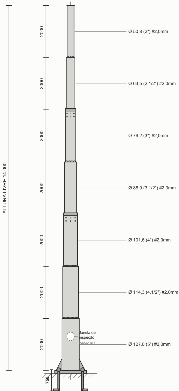
VISTA LATERAL — FLANGEADO medidas em mm
