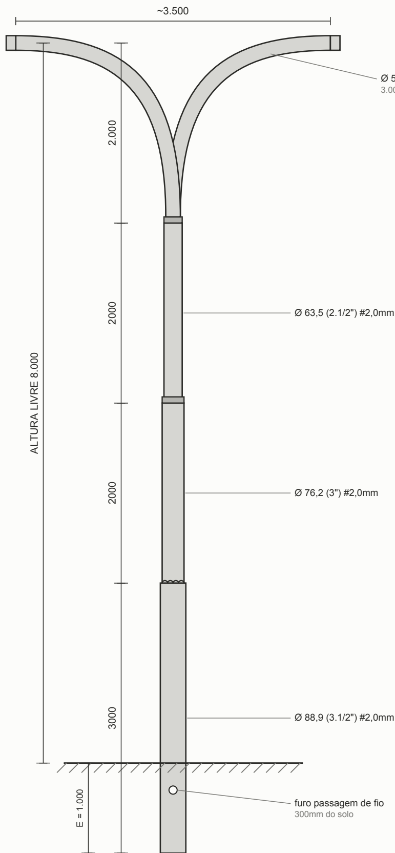
VISTA LATERAL — ENGASTADO
