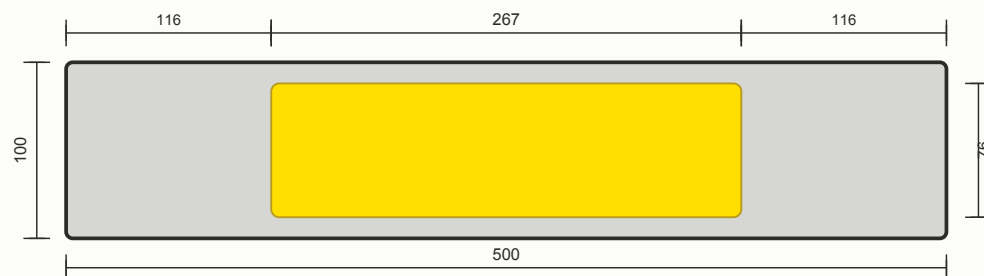
VISTA INFERIOR — FACE DO LED (corte a laser)
