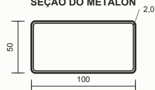
SEÇÃO DO METALON
