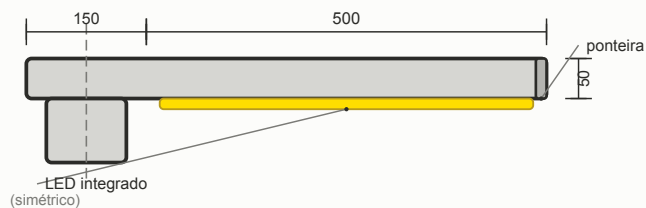
DETALHE DA CABEÇA
