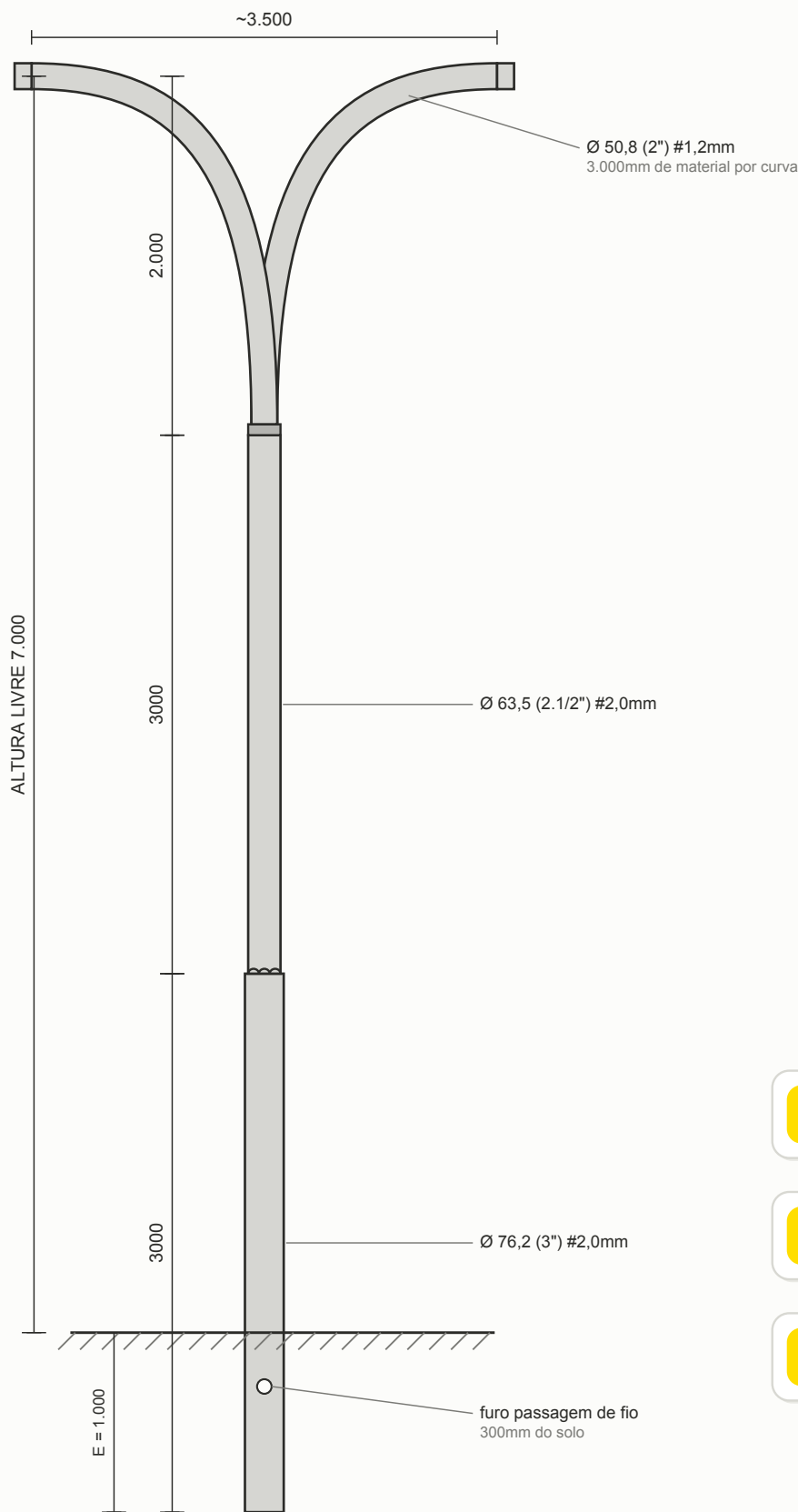
EMENDA MÓVEL encaixe de 150mm com luva interna 6 parafusos sextavados — espaçamento 120°
