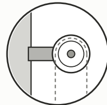
ROLDANA 2.1/2" canal "V" — suporte lateral chapa 5×3 corda de içamento passa no canal
