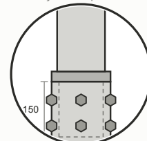
EMENDA MÓVEL encaixe de 150mm com luva interna 6 parafusos sextavados — espaçamento 120°
