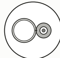
ARRUELA-GUIA · VISTA SUPERIOR \varnothing 125 mm deitada, soldada DIRETA ao tubo corda passa por dentro — de lado é só um traço
