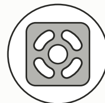
SAPATA / FLANGE placa 280 \times 280mm · chapa 1/2" furos oblongos em curva — nivelamento
