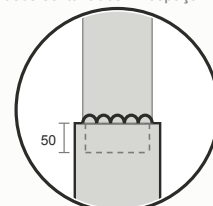
EMENDA FIXA encaixe de 50mm soldado solda circunferencial estrutural
