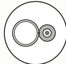
ARRUELA-GUIA · VISTA SUPERIOR Ø125mm deitada, soldada DIRETA ao tubo corda passa por dentro — de lado é só um traço
