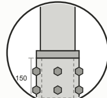
EMENDA MÓVEL encaixe de 150mm com luva interna 6 parafusos sextavados — espaçamento 120°
