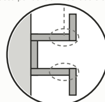
AMARRAÇÃO DA CORDA cleat em "U" c/ bordas — ferro chato 1"×1/8" base soldada no tubo — corda amarra em "8"
