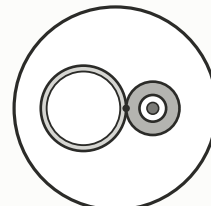
ARRUELA-GUIA · VISTA SUPERIOR Ø125mm deitada, soldada DIRETA ao tubo corda passa por dentro — de lado é só um traço
