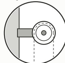
ROLDANA 2.1/2" canal "V" — suporte lateral chapa 5×3 corda de içamento passa no canal
